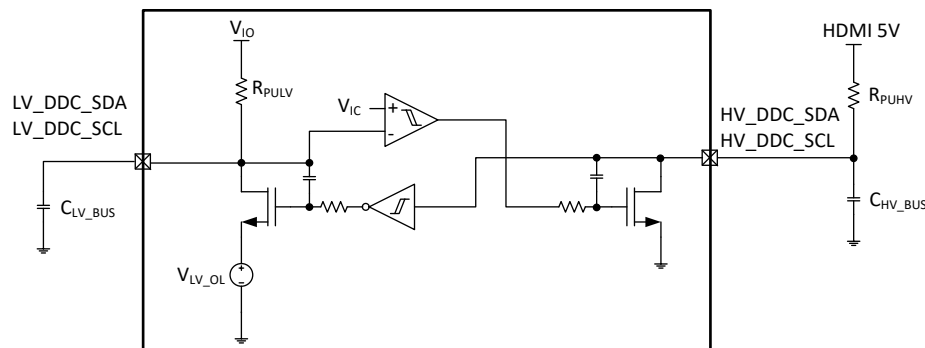
図 8-4. DDC Buffer Block Diagram
