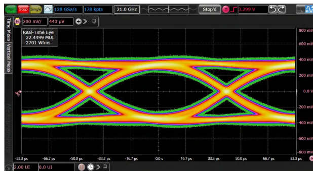
9-7. 12 Gbps Output Eye at TTP4 After Pre and Post Channels
