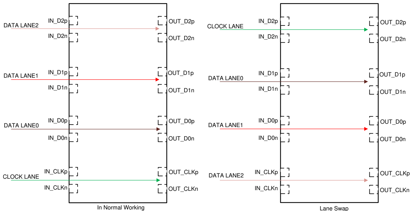
図 8-1. TDP1204 Swap Function
