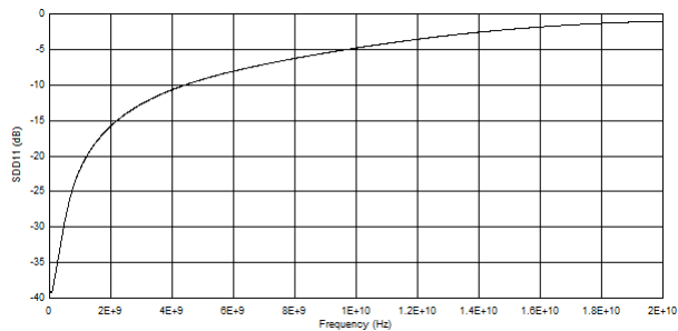
図 6-4. Input Differential Return Loss (SDD11)
