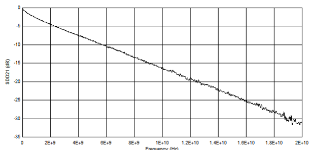
9-4. Pre-Channel Insertion Loss at TTP2
