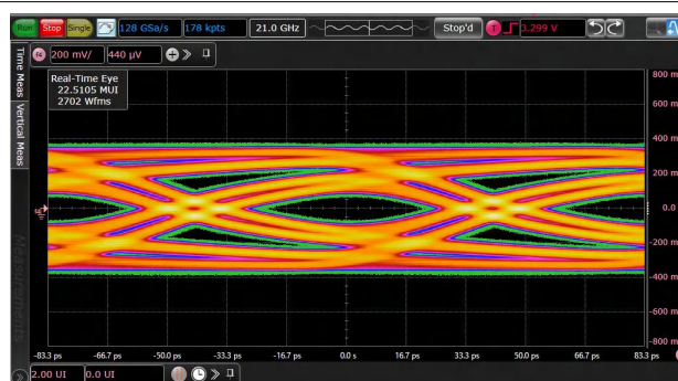
9-6. 12 Gbps Input Eye at TTP2 After Pre-channel
