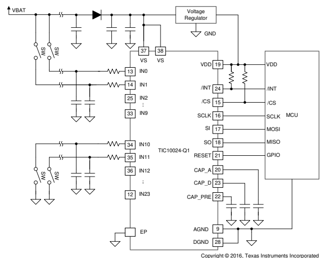
概略回路図
