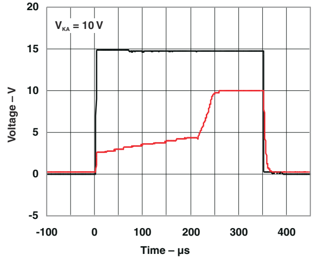
図 5-6. 大信号パルス応答
