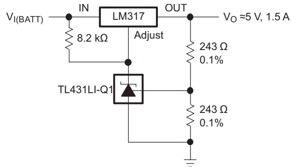
FIG 31. Precision 5-V, 1.5-A Regulator
