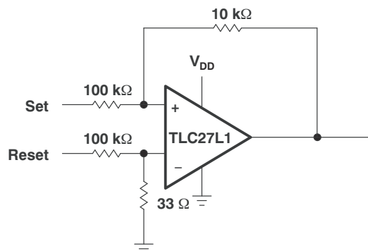
図 7-14. フリップフロップの設定/リセット
