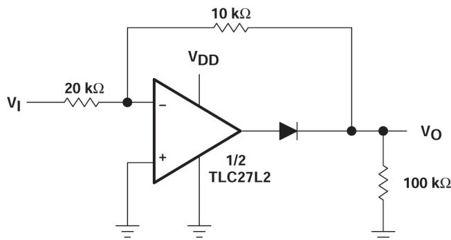
図 7-12. 全波整流器、 f_c = 1\text{kHz} および R_L = 10\text{k}\Omega に正規化
