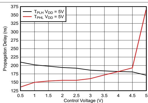
図 5-8. 伝搬遅延と制御電圧との関係
