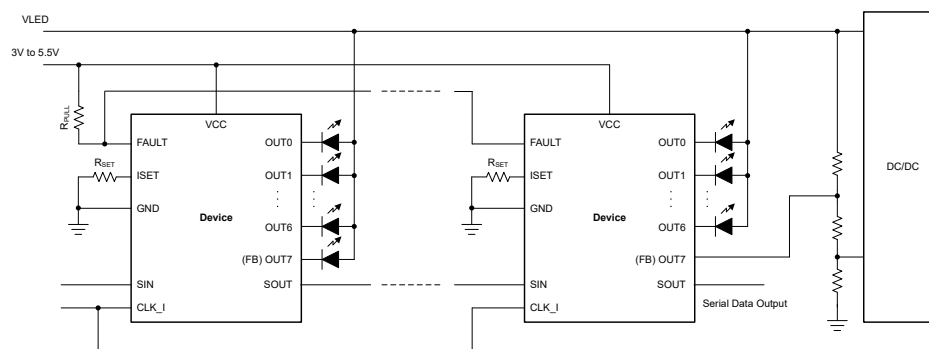
概略回路図
