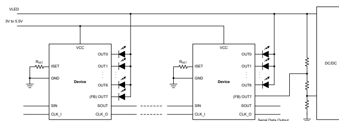
概略回路図
