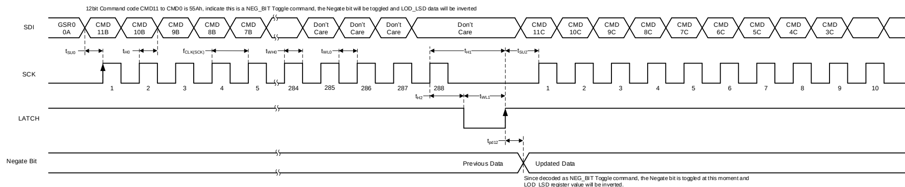
图 6. Negate Bit Toggle
