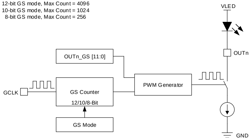
FIG 22. PWM Generator
