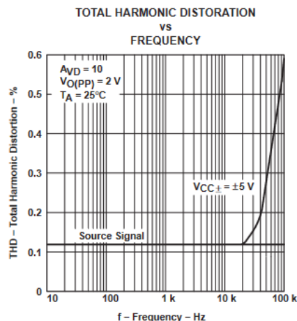
図 5-14. 全高調波歪と周波数との関係
