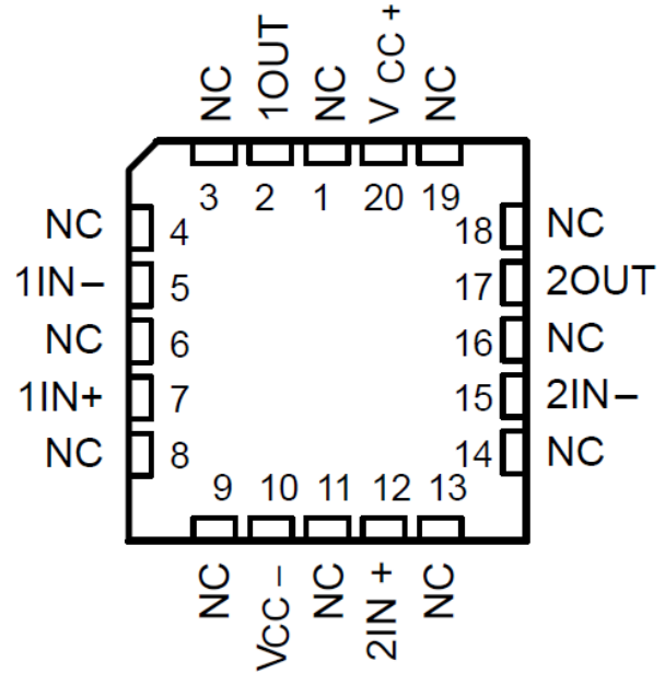
図 4-6. TLE2062M、TLE2062AM、TLE2062BM FK パッケージ (上面図)
