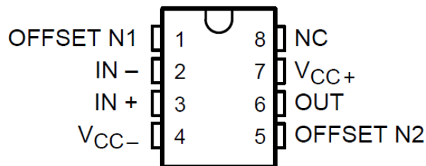
図 4-1. TLE2061M、TLE2061xM、JG パッケージ、(上面図)
