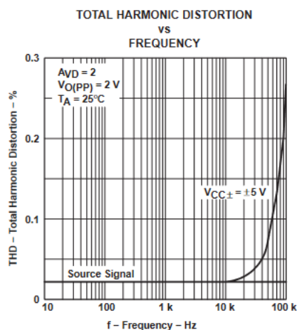
図 5-13. 全高調波歪と周波数との関係
