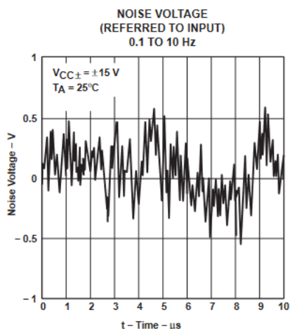
図 5-11. ノイズ電圧
