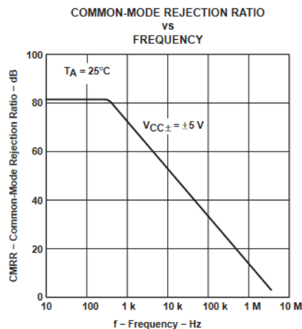
図 5-8. 同相除去比と周波数との関係
