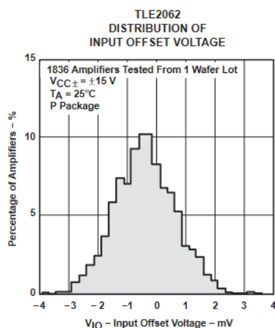
図 5-2. TLE2062 入力オフセット電圧の分布
