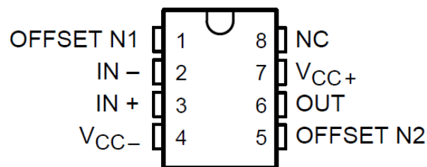
図 4-1. TLE2061M、TLE2061xM、JG パッケージ、(上面図)
