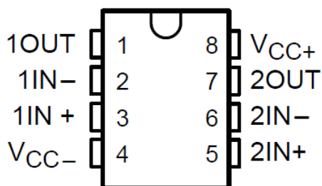
図 4-3. TLE2062、TLE2062A、TLE2062B D、JG、または P パッケージ (上面図)
