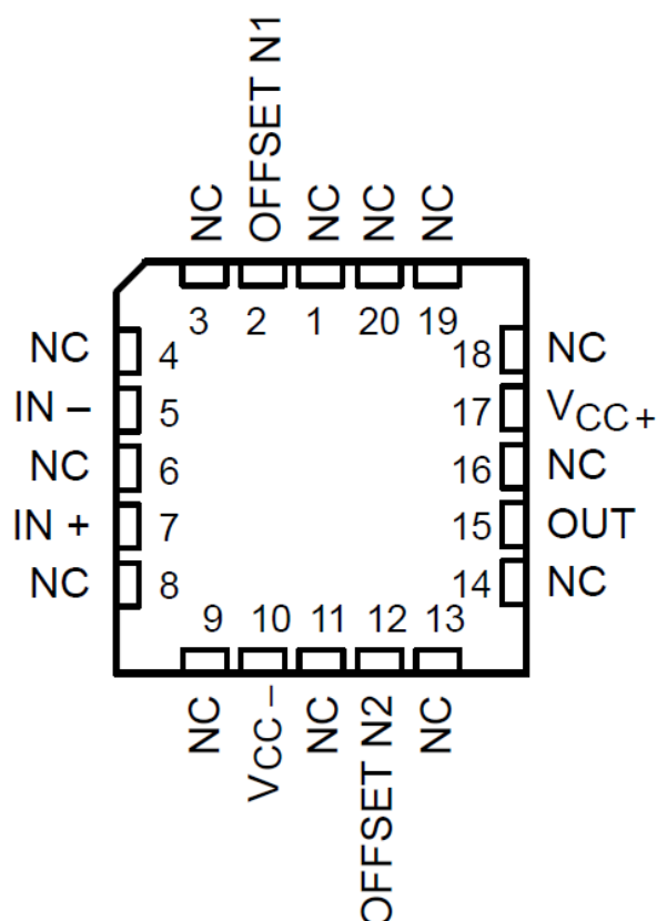
図 4-5. TLE2061M、TLE2061AM、TLE2061BM FK パッケージ (上面図)
