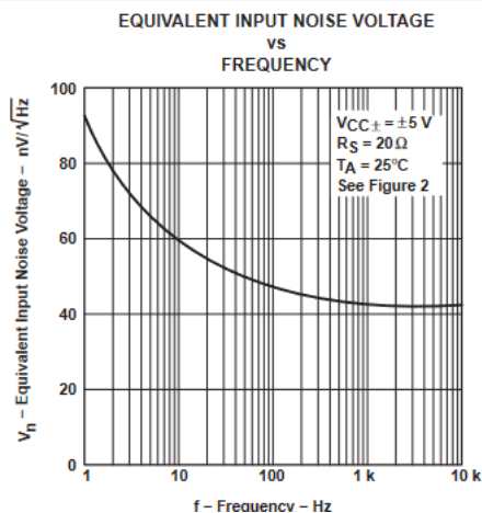
図 5-12. 等価入力ノイズ電圧と周波数との関係
