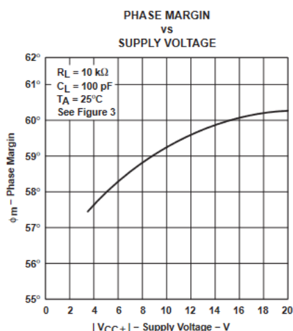
図 5-15. 位相マージンと電源電圧との関係
