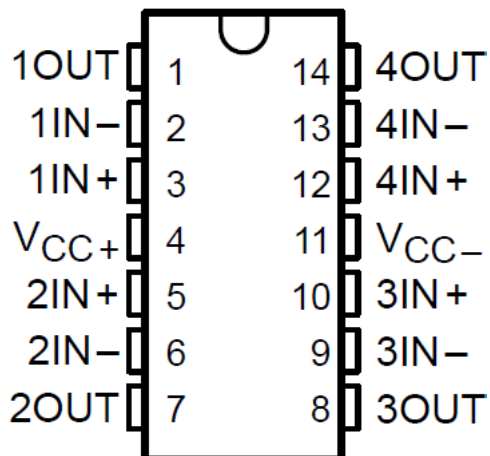
図 4-4. TLE2064、TLE2064A、および TLE2064B D、J、N、または W パッケージ (上面図)
