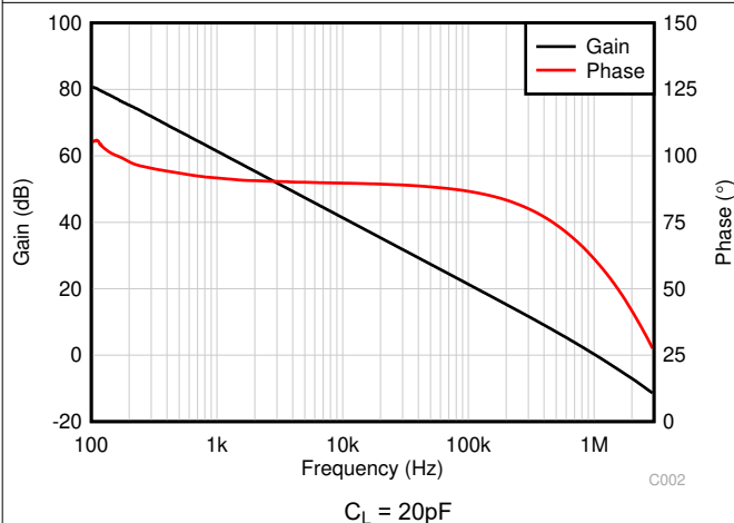
図 5-17. 開ループ ゲインおよび位相と周波数との関係
