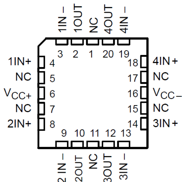
図 4-7. TLE2064M、TLE2064AM、TLE2064BM FK パッケージ (上面図)
