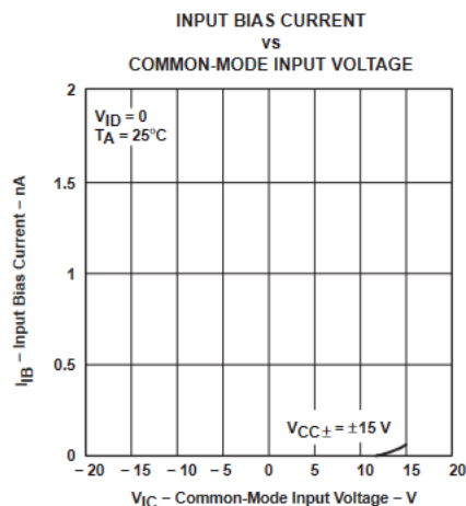
図 5-4. 入力バイアス電流と同相入力電圧との関係
