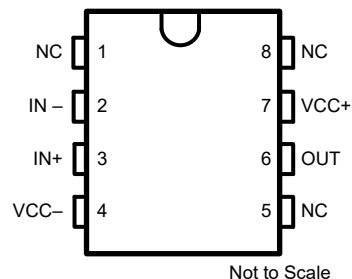
図 4-2. TLE2061、TLE2061A、D、P パッケージ、(上面図)
