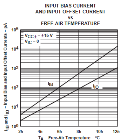
図 5-5. 入力バイアス電流および入力オフセット電流と自由気流での周囲温度との関係
