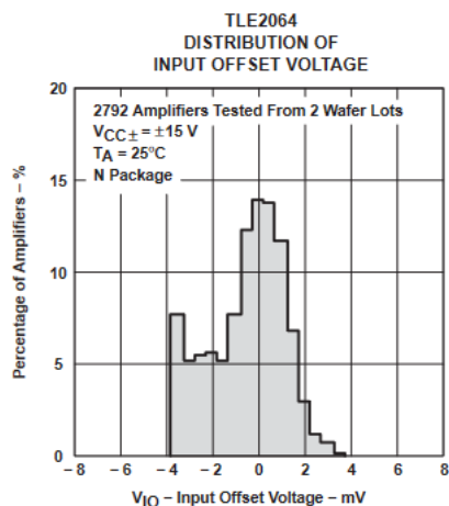
図 5-3. TLE2064 入力オフセット電圧の分布
