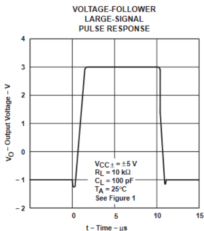
図 5-9. 電圧フォロワの大信号パルス応答
