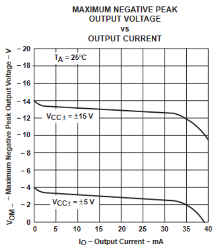
図 5-7. 最大負ピーク出力電圧と出力電流との関係
