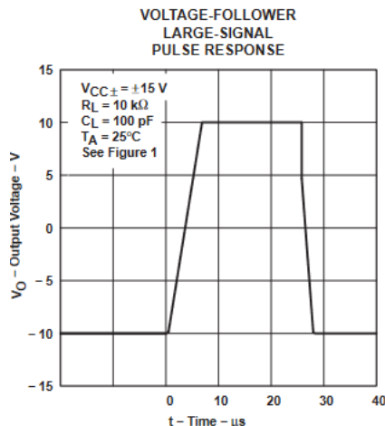
図 5-10. 電圧フォロワの大信号パルス応答
