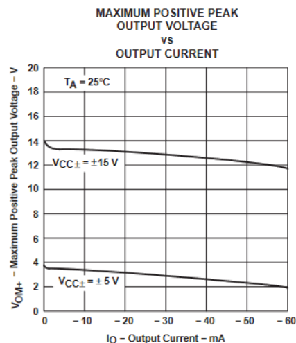
図 5-6. 最大正ピーク出力電圧と出力電流との関係
