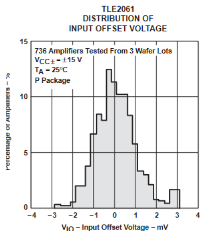
図 5-1. TLE2061 入力オフセット電圧の分布
