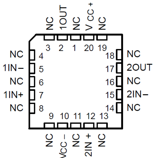
図 4-6. TLE2062M、TLE2062AM、TLE2062BM FK パッケージ (上面図)
