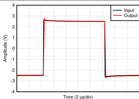
図 6-13. 小信号パルス応答
