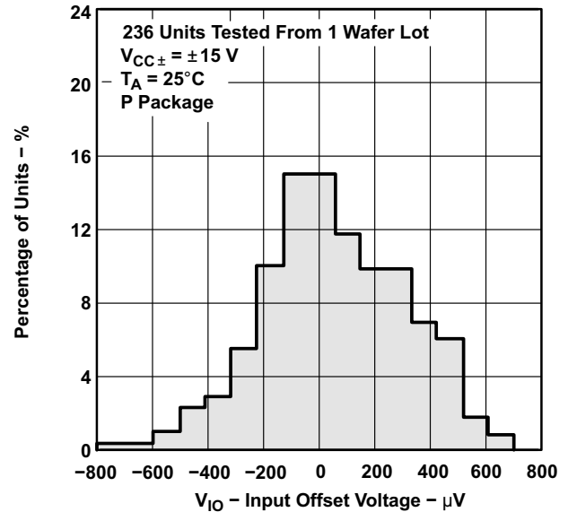
図 5-2. TLE2142 入力オフセット電圧の分布
