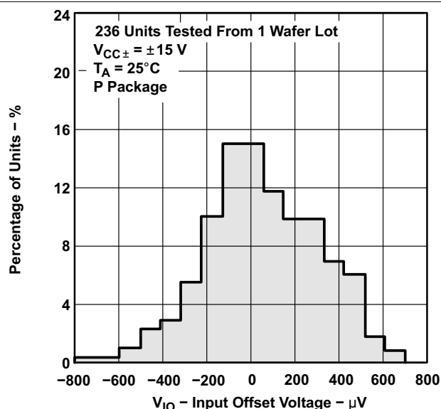
図 5-2. TLE2142 入力オフセット電圧の分布
