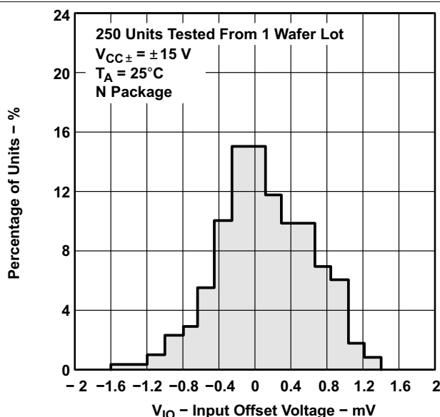
図 5-1. TLE2141 入力オフセット電圧の分布
