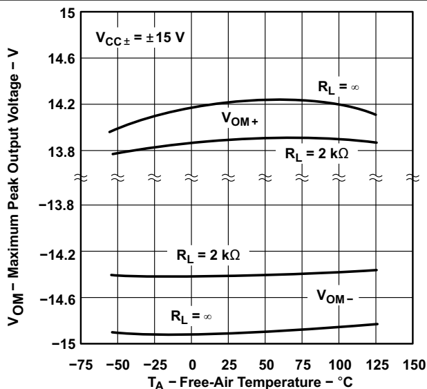
図 5-8. 最大ピーク出力電圧と自由気流温度との関係
