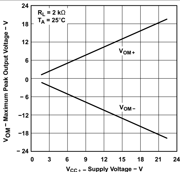
図 5-7. 最大ピーク出力電圧と電源電圧との関係
