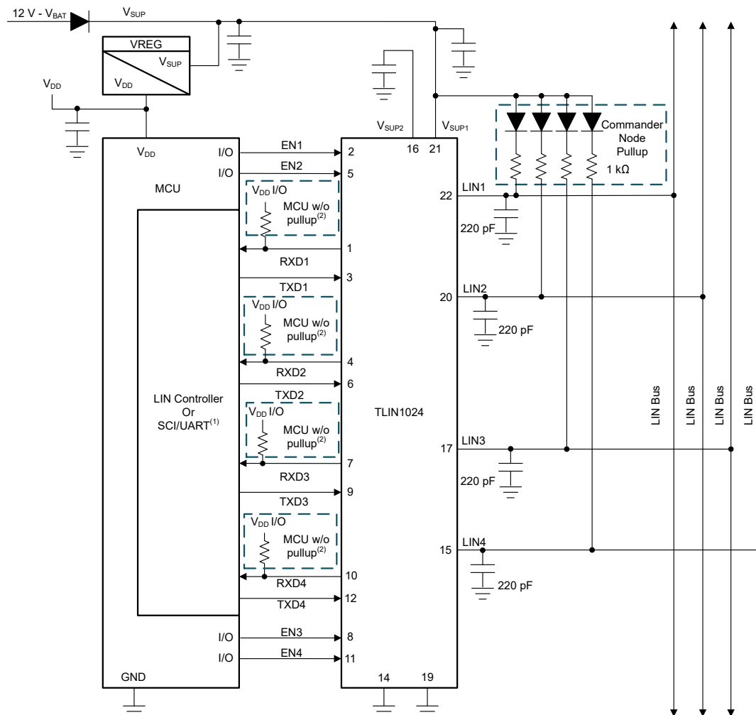
図 8-1. Typical LIN Bus
