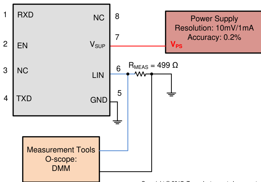
図 6-7. I_{BUS\_PAS\_DOM} のテスト回路：TXD = リセツプ状態、 V_{BUS} = 0V 、パラメータ 13
