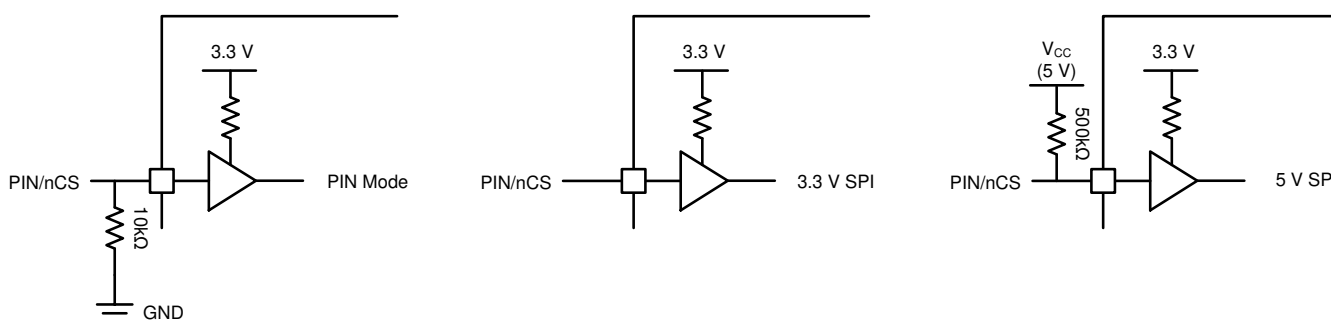
图 9-4. PIN/nCS Configuration
