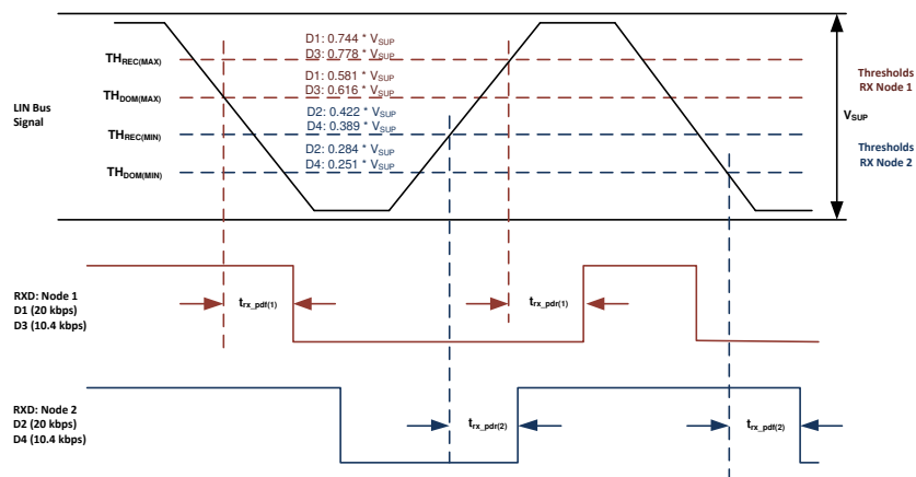
図 6-4. 伝搬遅延
