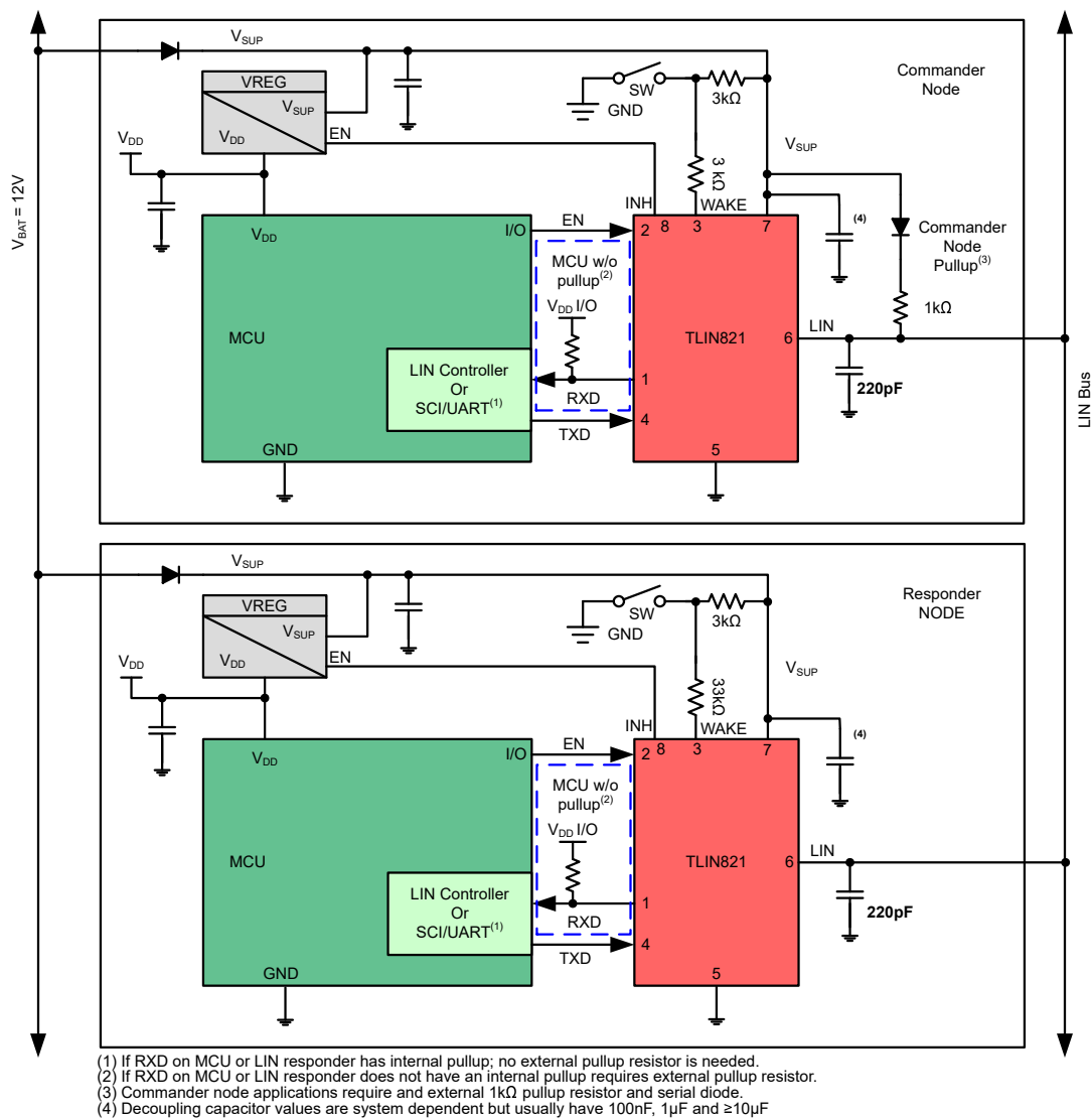
図 8-1. 代表的な LIN バス
