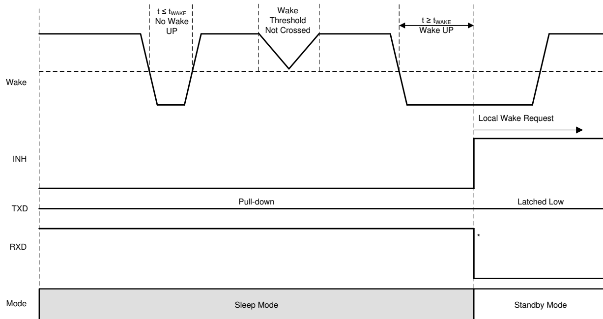
図 7-6. ローカル ウェークアップ - 立ち下がりエッジ
