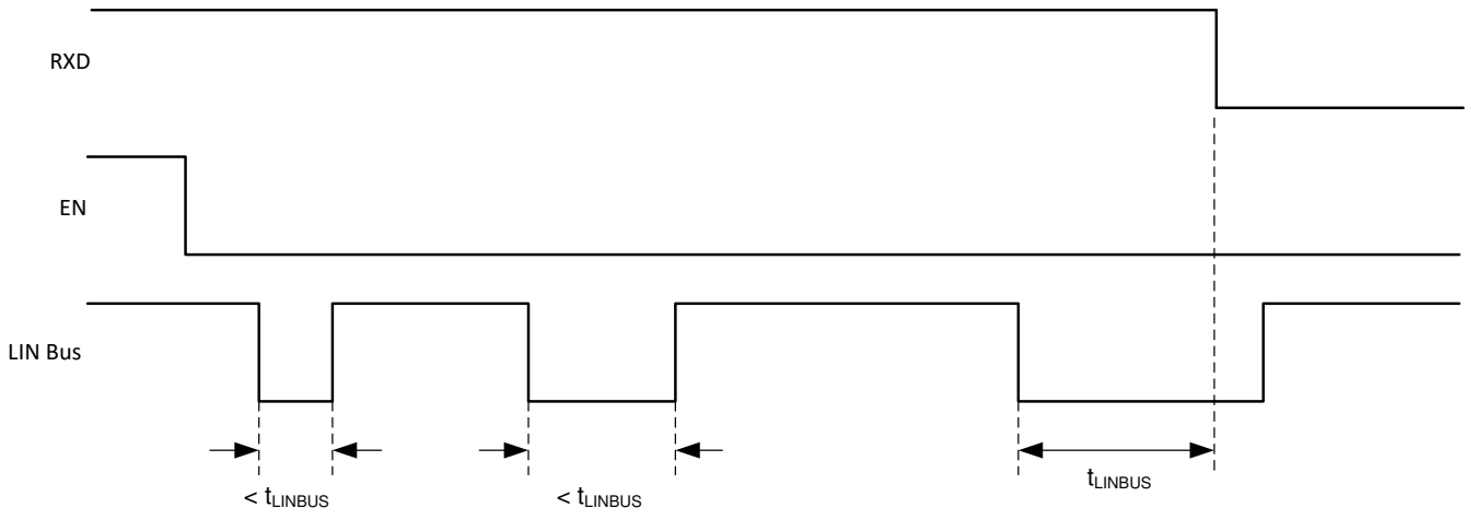
図 7-2. バス フォルトなし：バス リセッス条件とウェイクアップによるスリープモードへの移行
