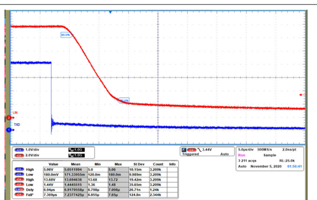
図 8-3. リセッティングからドミナントまでの伝搬遅延
