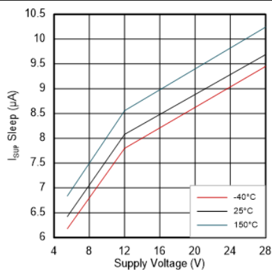
図 5-1. スリープモード I_{SUP} と V_{SUP} および温度との関係
