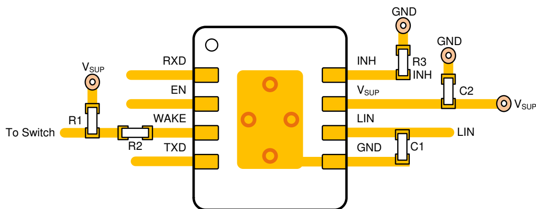
図 8-4. レイアウト例
