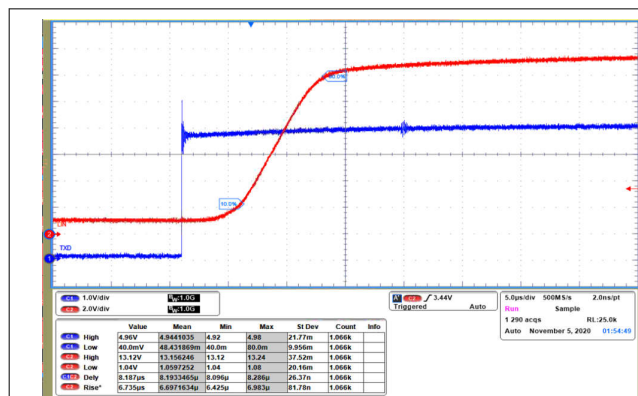
図 8-2. ドミナントからリセッティングまでの伝搬遅延
