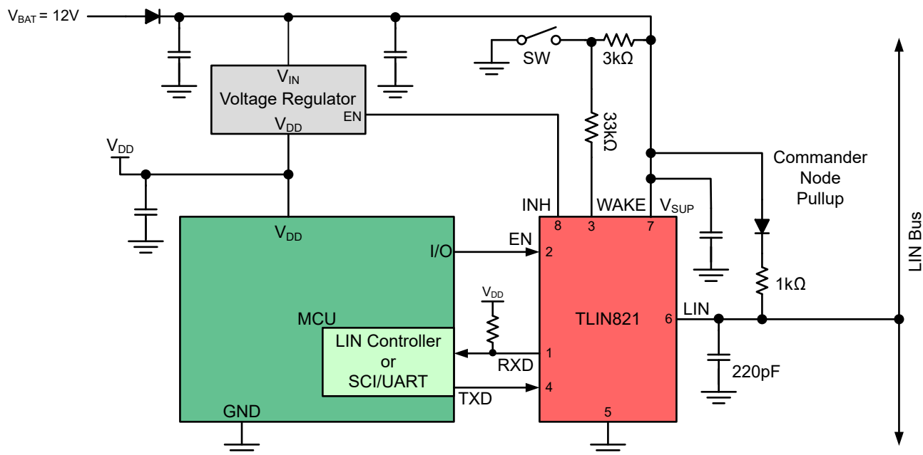
コマンダ ノードの概略回路図
