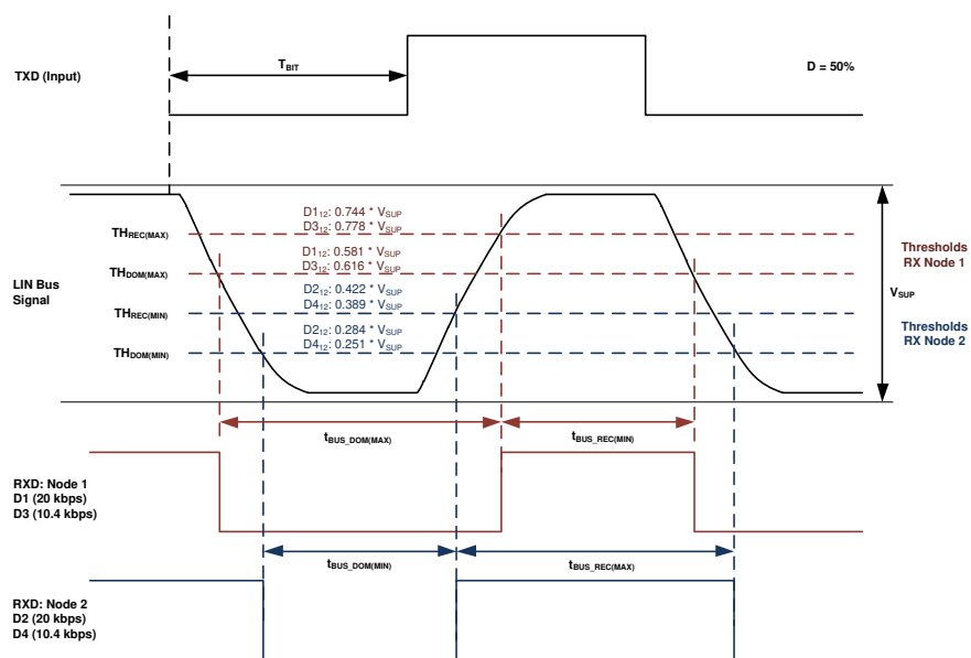
図 6-3. バス タイミング パラメータの定義
