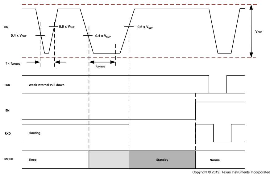
図 6-7. LIN によるウェークアップ
