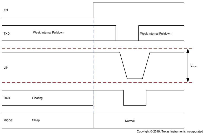
図 6-6. EN によるウェークアップ
