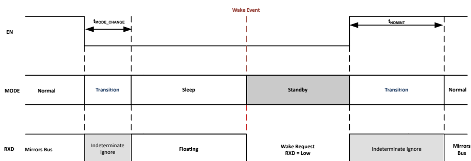
図 6-5. モード遷移
