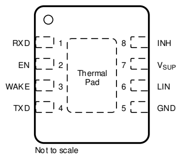
図 4-2. DRB パッケージ、8 ピン (VSON) 上面図
