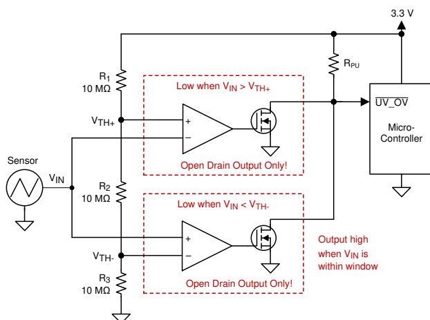
図 7-7. Window Comparator
