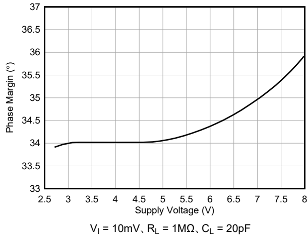
図 5-31. 位相マージンと電源電圧との関係
