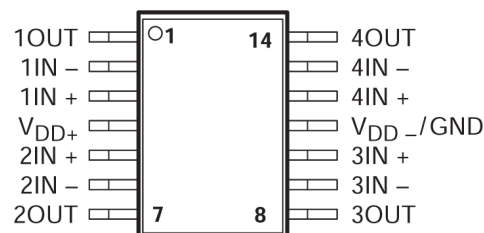
図 4-3. TLV2324 D パッケージ、14 ピン SOIC、または N パッケージ、14 ピン PDIP (上面図)
