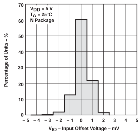
図 5-4. TLV2324 入力オフセット電圧の分布
