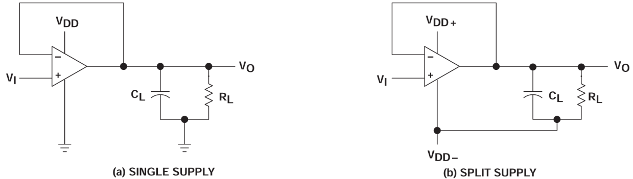
図 6-1. ユニティ ゲイン アンプ
