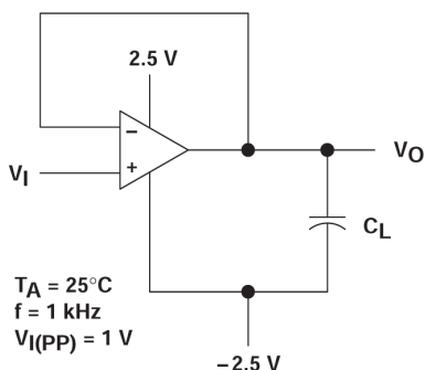
図 7-7. 出力特性のテスト回路
