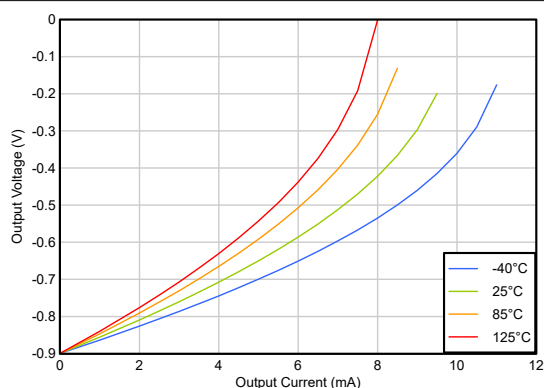
図 5-23. 出力電圧スイングと 出力電流との関係 (シンク)
