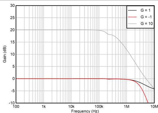
図 5-19. 開ループ ゲインと周波数との関係
