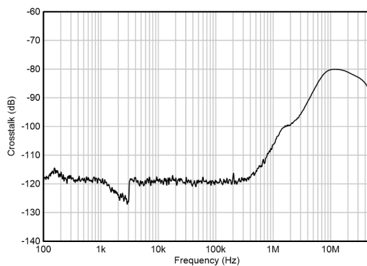
図 5-49. チャネル セパレーション
