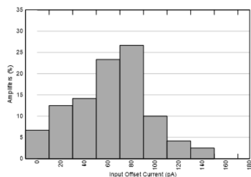
図 5-10. 入力オフセット電流の分布
