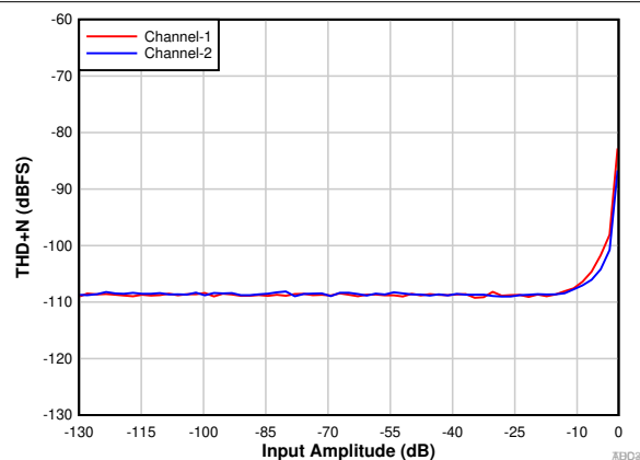
图 9-3. THD+N vs Input Amplitude
