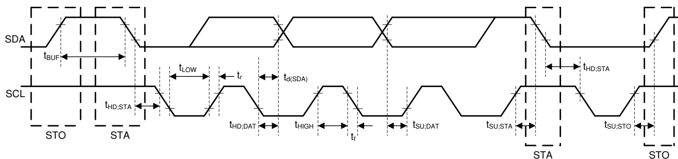
图 7-1. I²C Interface Timing Diagram
