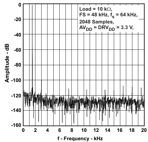
8-12. Right ADC FFT
