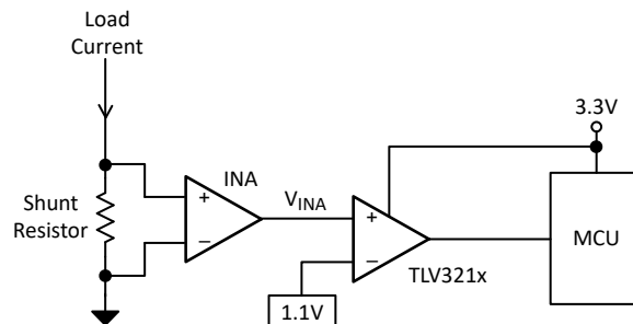
図 7-7. 電流検出
