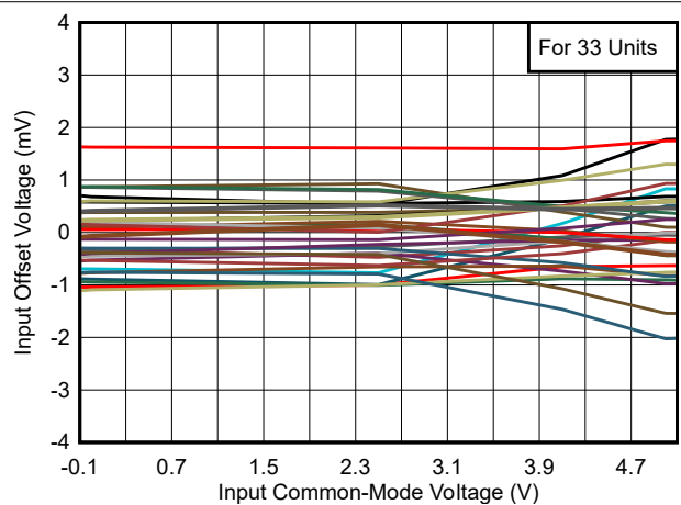
図 5-5. オフセットと同相との関係、5V
