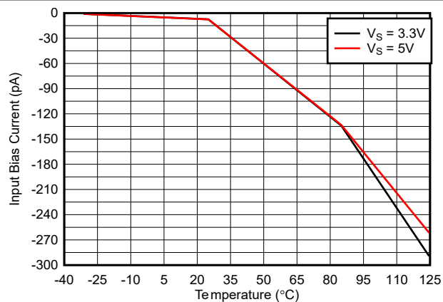
図 5-8. バイアス電流と温度との関係
