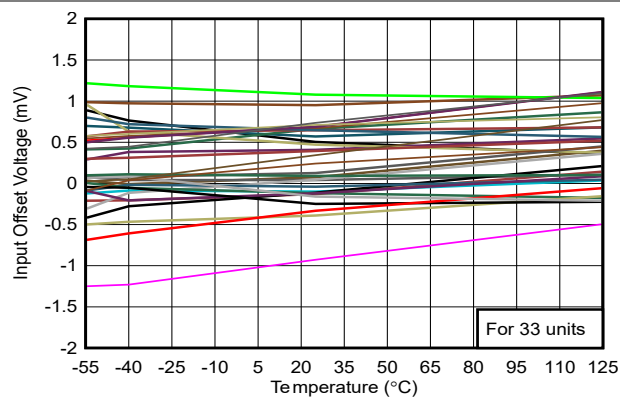
图 5-3. Offset vs. Temperature
