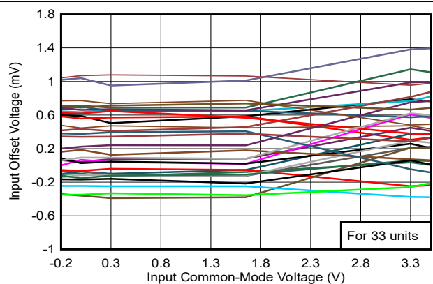
图 5-7. Offset vs. Common-Mode, 3.3V
