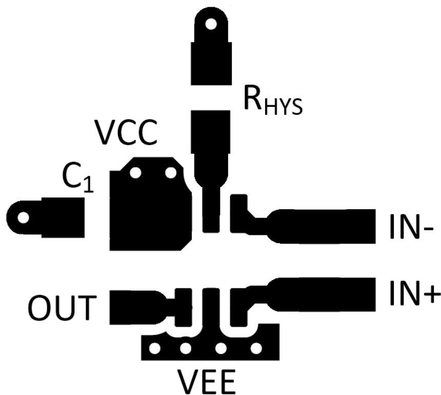
図 9-1. TLV3603-EP Layout Example
