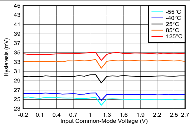
图 5-6. Hysteresis vs. Common-Mode, 2.5V
