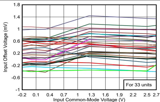
图 5-5. Offset vs. Common-Mode, 2.5V
