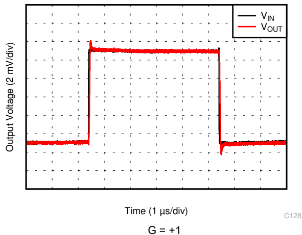
図 5-24. 小信号ステップ応答
