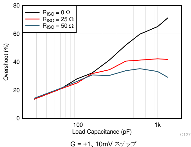
図 5-20. 小信号オーバーシュートと容量性負荷との関係
