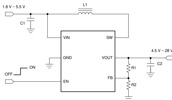
概略回路図
