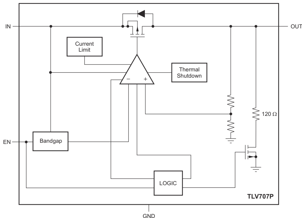
图 7-2. TLV707P Block Diagram
