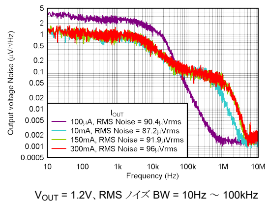
図 5-18. ノイズ
