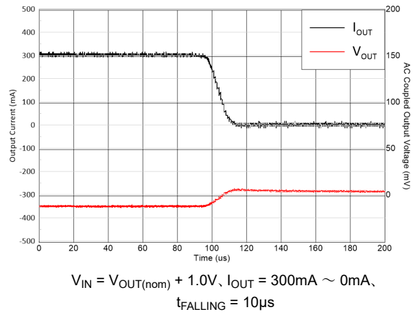
図 5-14. 負荷過渡
