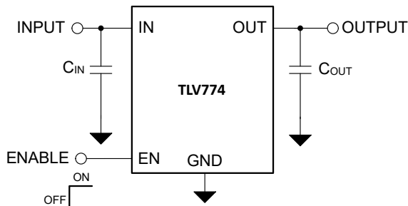
図 7-1. TLV774 の代表的なアプリケーション
