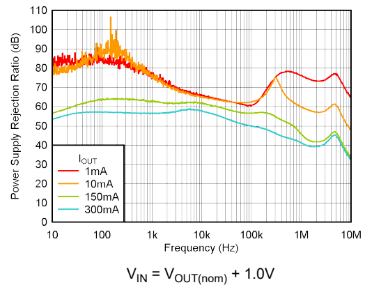
図 5-16. PSRR と周波数との関係
