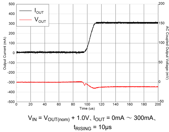
図 5-13. 負荷過渡
