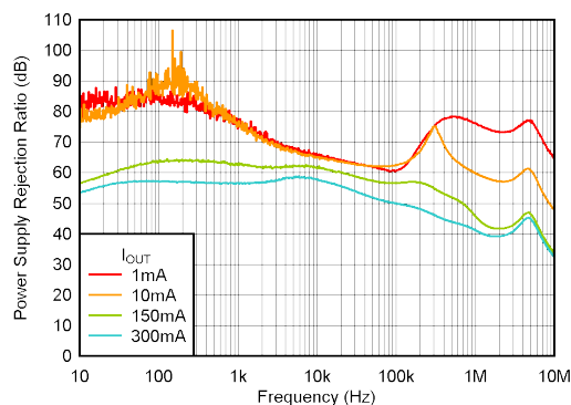
図 7-3. PSRR
