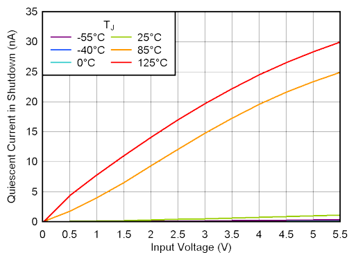
図 5-7. 静止電流と V_{IN} との関係
