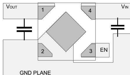
図 7-4. DQN パッケージ (X2SON) の標準レイアウト
