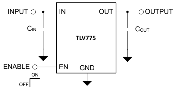
図 7-1. TLV775 の代表的なアプリケーション
