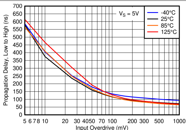
図 5-22. 伝搬遅延、"Low" から "High", 5V
