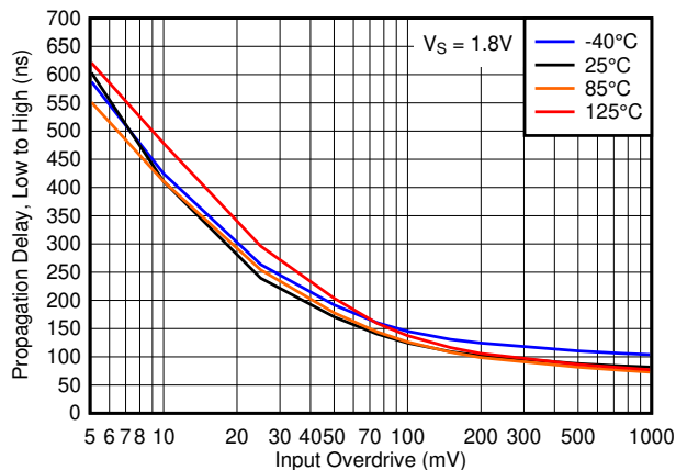
図 5-18. 伝搬遅延、"Low" から "High", 1.8V
