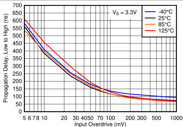
図 5-20. 伝搬遅延、"Low" から "High", 3.3V
