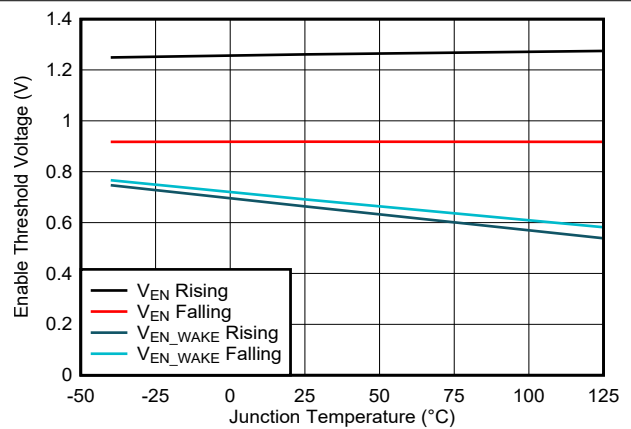
図 7-6. イネーブル・スレッショルド
