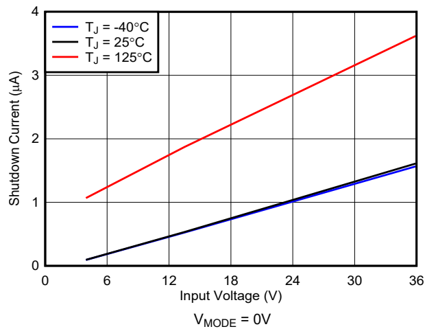
図 7-1. シャットダウン時の電源電流
