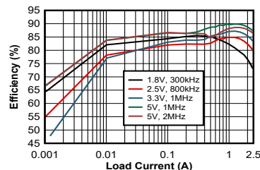
効率と出力電流との関係 ( V_{IN} = 24\text{V} )
