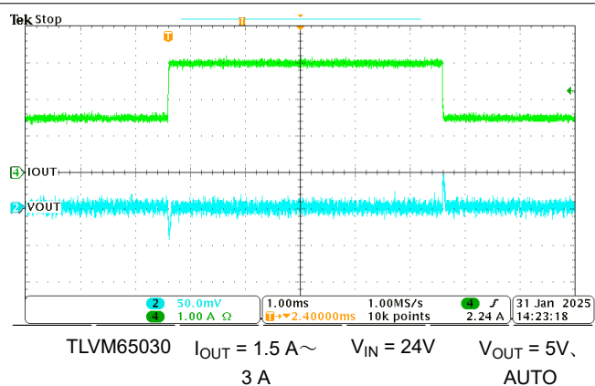
図 7-6. 負荷過渡 (50% ~ 100%)
