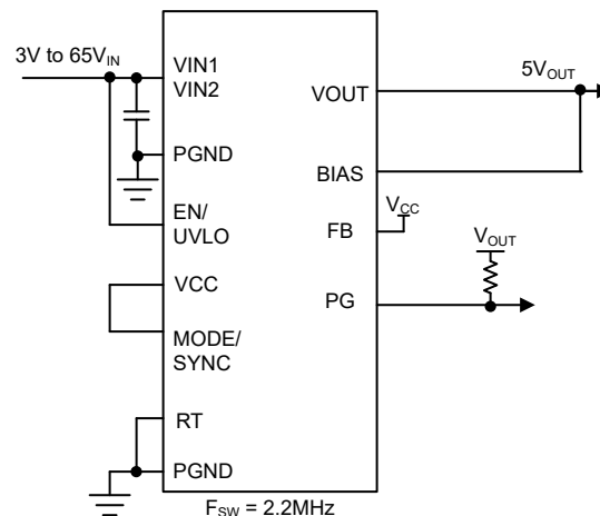
概略回路図
