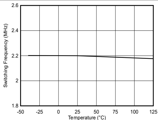
図 5-5. f_{SW} 2.2MHz
