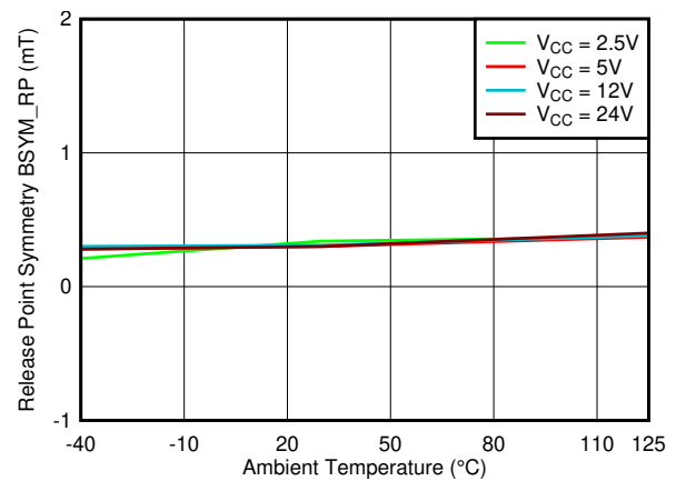
図 6-32. B_{SYM\_RP(ZY)} vs Temperature
