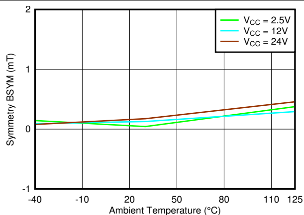
図 6-58. B_{SYM(Z)} vs Temperature
