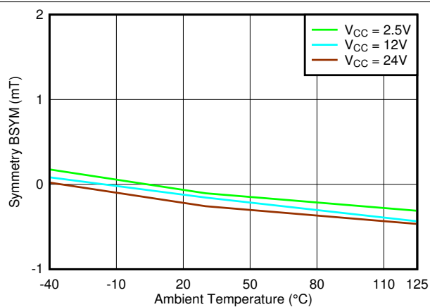
図 6-60. B_{SYM(X)} vs Temperature
