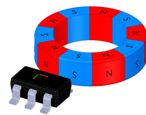
図 7-6. XY Outer Edge 2
