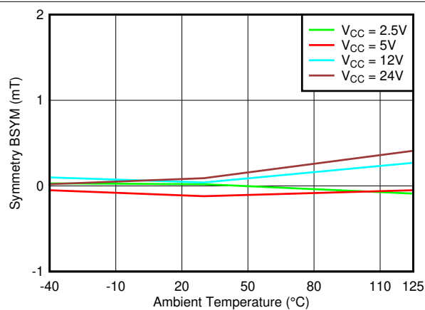
図 6-22. B_{SYM(X)} vs Temperature
