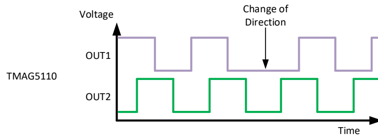
図 8-2. TMAG5110-Q1 Output Response
