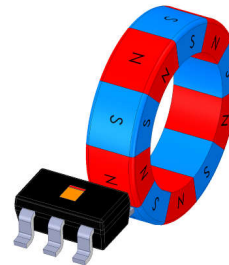
図 7-10. ZY Outer Edge 1
