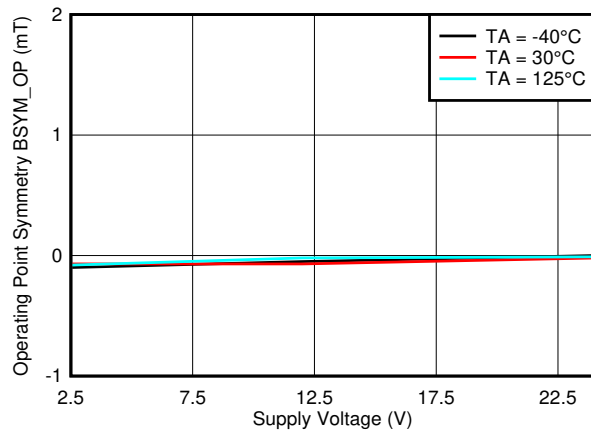
図 6-33. B_{SYM\_OP(XY)} vs V_{CC}
