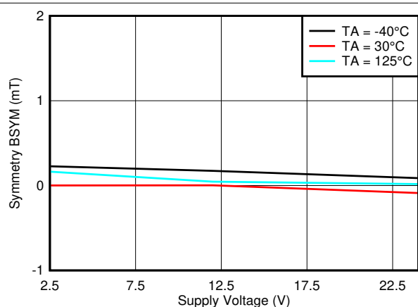
図 6-61. B_{SYM(Y)} vs V_{CC}
