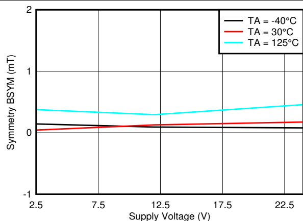
図 6-57. B_{SYM(Z)} vs V_{CC}
