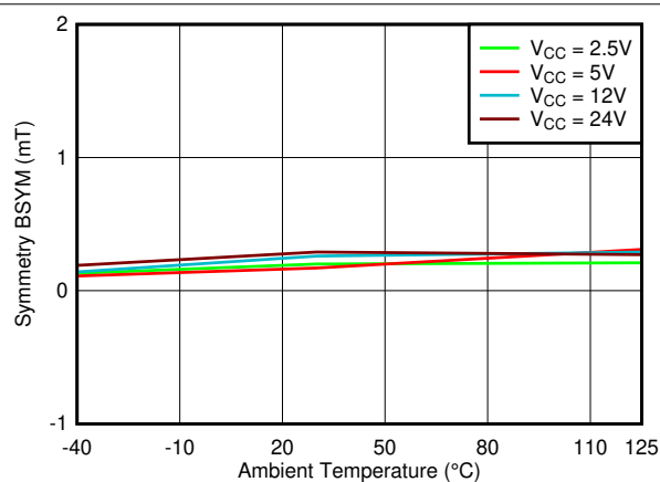
図 6-24. B_{SYM(Y)} vs Temperature
