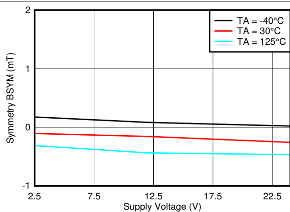
図 6-59. B_{SYM(X)} vs V_{CC}
