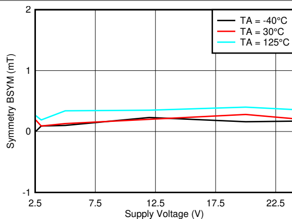
図 6-19. B_{SYM(Z)} vs V_{CC}
