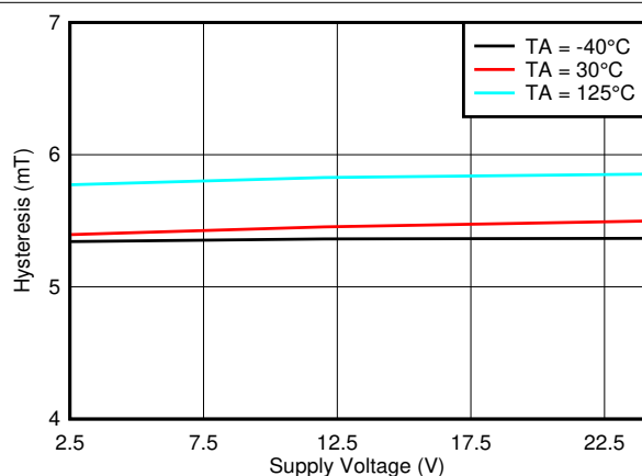
図 6-55. Hysteresis_Y vs V CC
