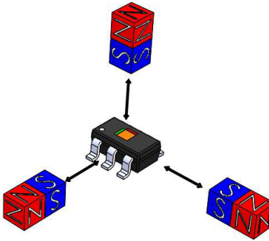
図 7-4. Axis Polarities
