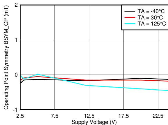
図 6-25. B_{SYM\_OP(ZX)} vs V_{CC}
