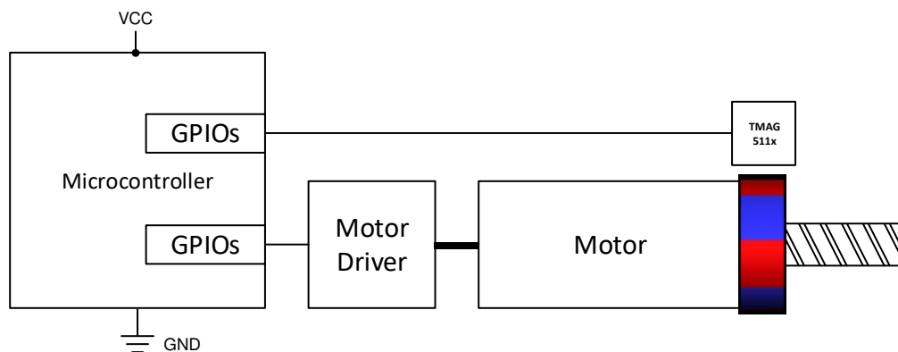
図 8-1. Incremental Encoding
