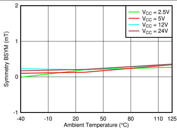
図 6-20. B_{SYM(Z)} vs Temperature
