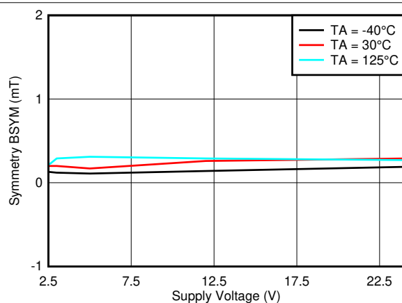
図 6-23. B_{SYM(Y)} vs V_{CC}
