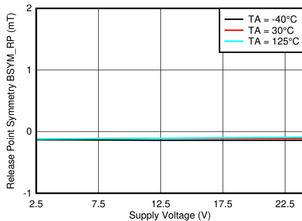
図 6-35. B_{SYM\_RP(XY)} vs V_{CC}
