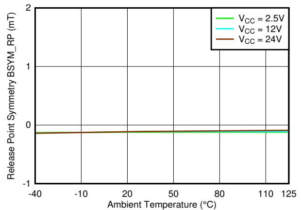
図 6-36. B_{SYM\_RP(XY)} vs Temperature
