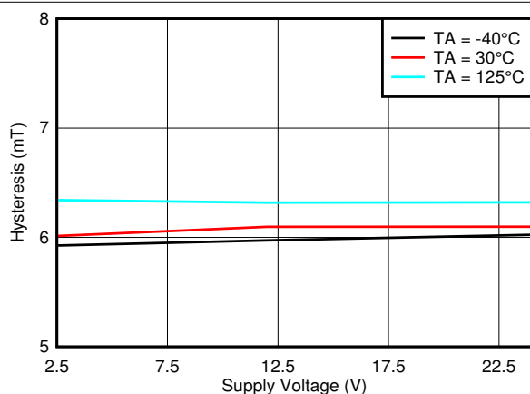
図 6-49. Hysteresis_X vs V CC
