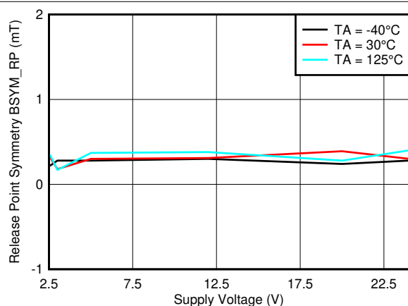
図 6-27. B_{SYM\_RP(ZX)} vs V_{CC}
