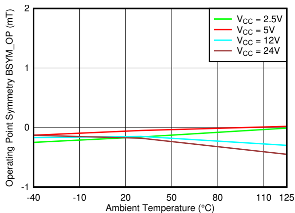
図 6-26. B_{SYM\_OP(ZX)} vs Temperature
