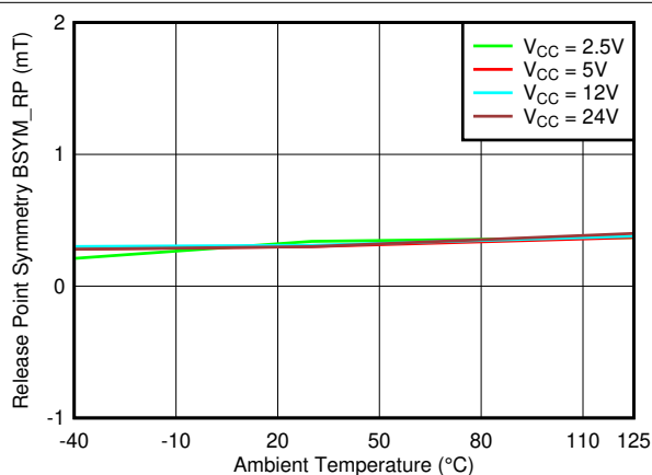
図 6-28. B_{SYM\_RP(ZX)} vs Temperature
