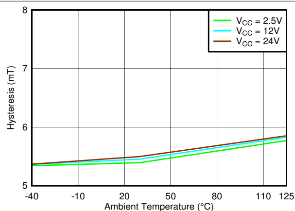
図 6-56. Hysteresis_Y vs Temperature
