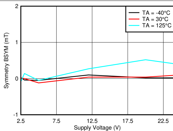
図 6-21. B_{SYM(X)} vs V_{CC}
