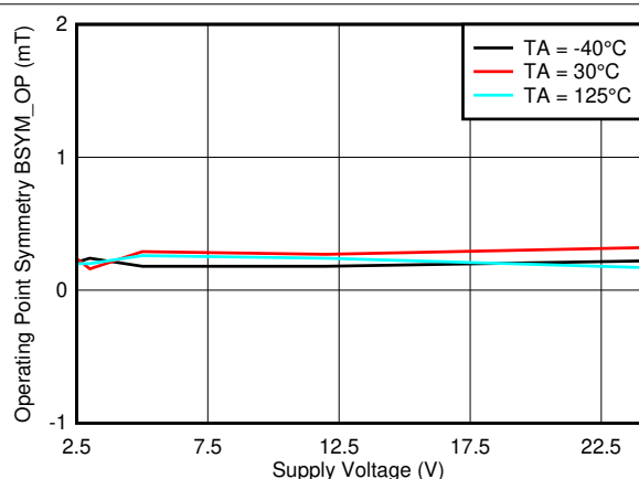
図 6-29. B_{SYM\_OP(ZY)} vs V_{CC}
