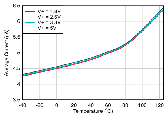
図 6-12. 平均静止電流と温度との関係
