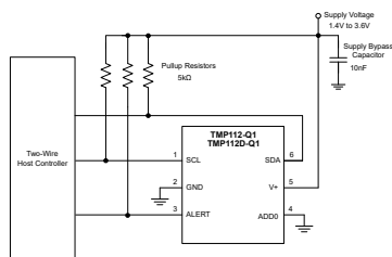
概略回路図 (SOT563 パッケージ)
