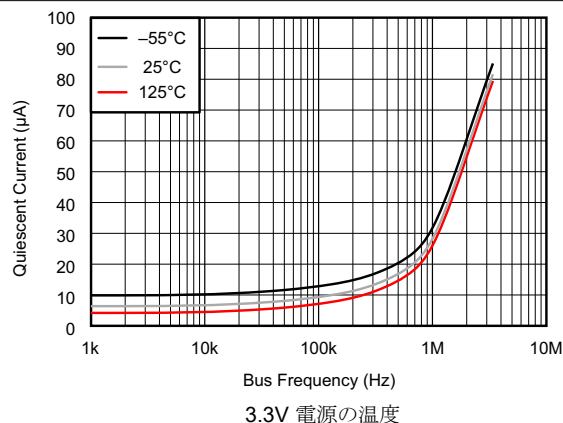
図 6-7. 静止電流とバス周波数との関係
