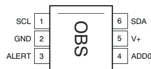
図 5-2. DRL パッケージ 6 ピン SOT563 TMP112D-Q1 および TMP112-Q1 (上面図)
