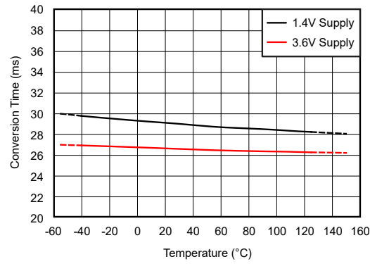
図 6-8. 変換時間と温度との関係
