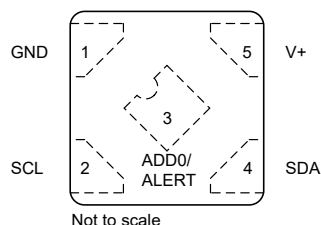
図 5-1. DPW パッケージ 5 ピン X2SON TMP112D-Q1 (上面図)
