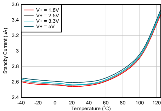
図 6-15. スタンバイ電流と温度との関係
