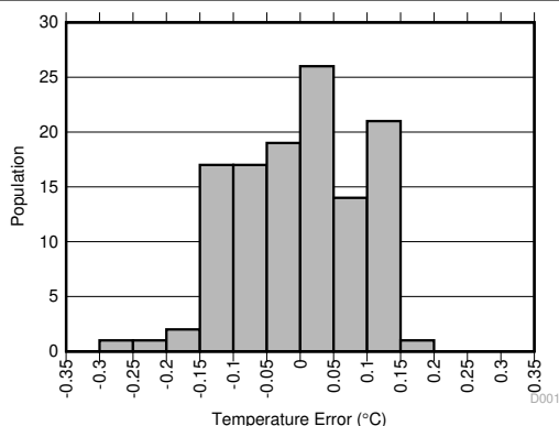
図 6-2. 25 °Cでの温度誤差
