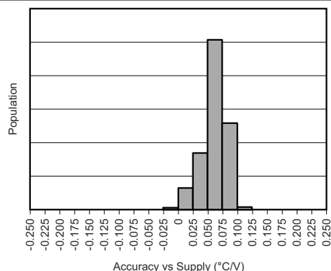
図 6-3. 精度と電源電圧との関係
