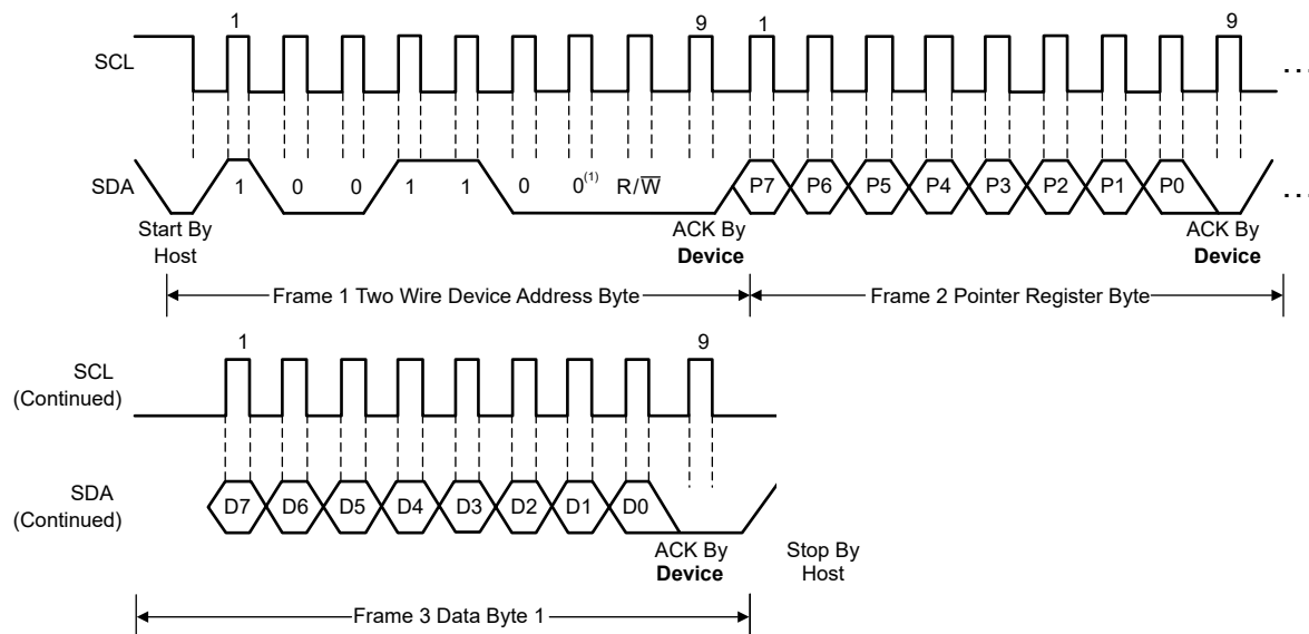
図 7-6. ワード形式書き込みでの 2 線式タイミング図
