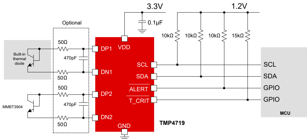
図 9-1. 設計例
