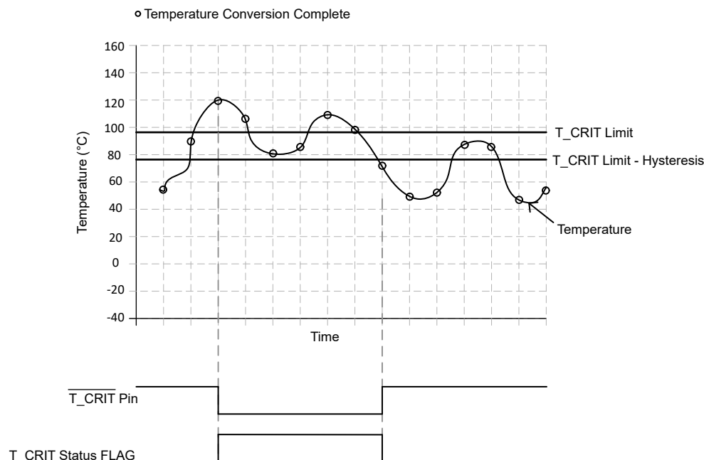
図 7-8. \overline{T\_CRIT} 出力タイミング図 — コンパレータ モード
