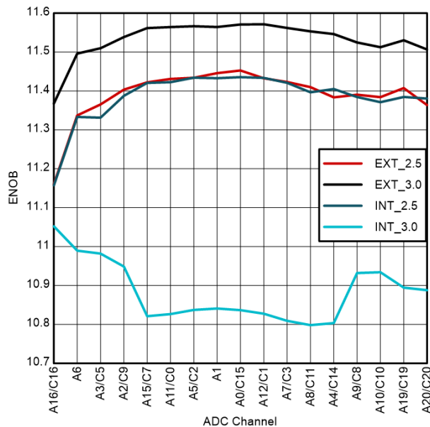
図 6-43. 48 ピン RGZ VQFN のチャンネルごとの ENOB
