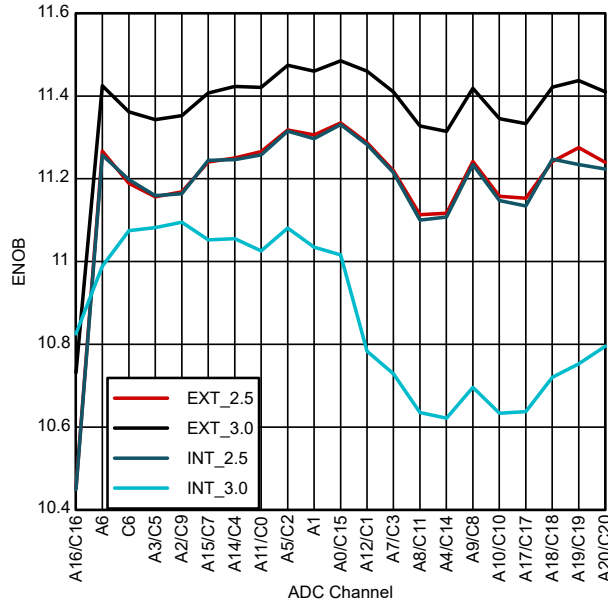
図 6-41. 64 ピン PM LQFP のチャンネルごとの ENOB
