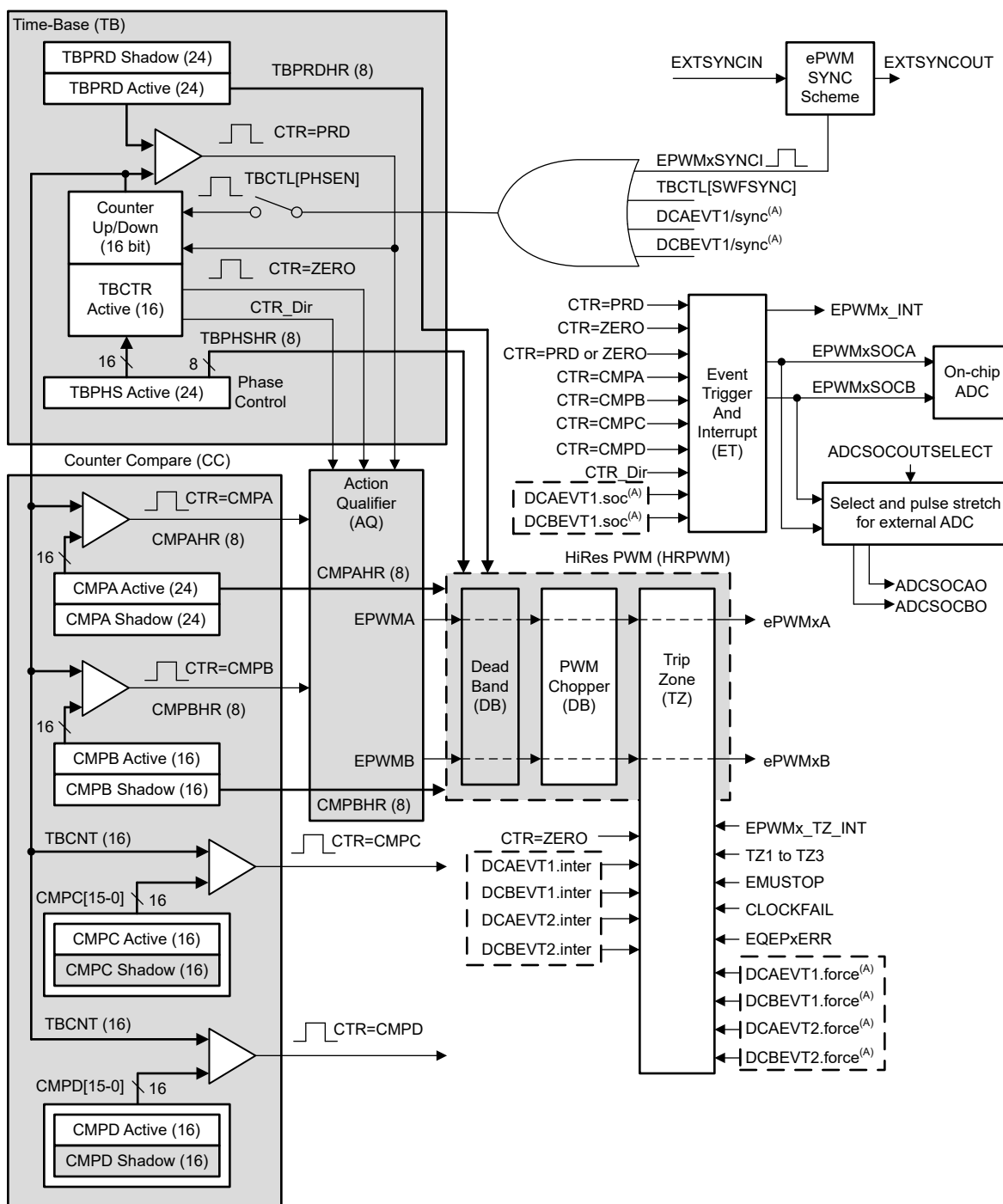
図 6-55. ePWM サブモジュールおよび重要な内部信号の相互接続
