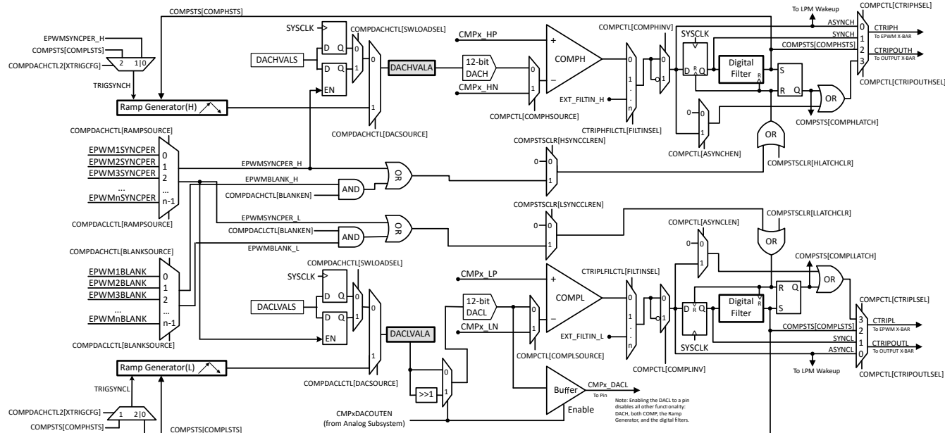
図 6-46. CMPSS モジュールのブロック図
