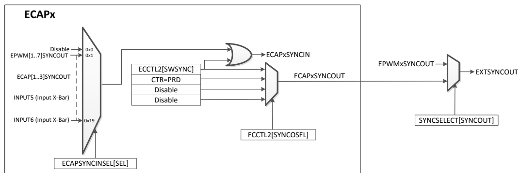
図 6-56. eCAPsynchronization 方式
