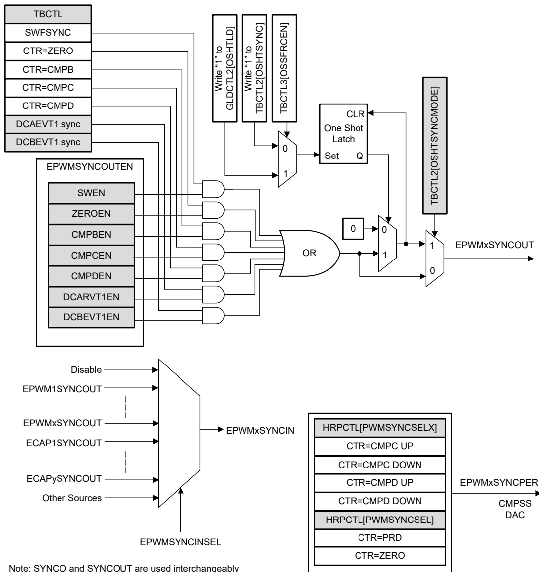
図 6-52. 同期チェーンのアーキテクチャ
