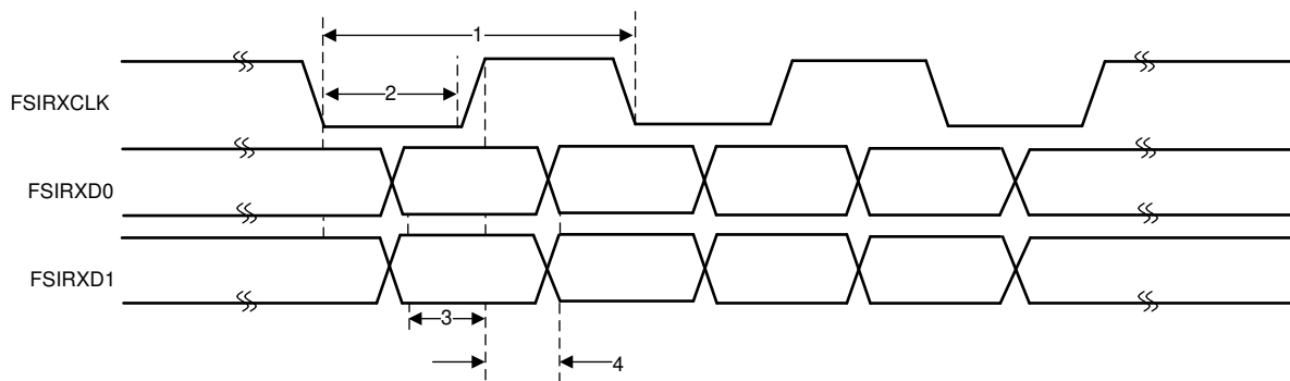
図 6-76. FSIRX タイミング
