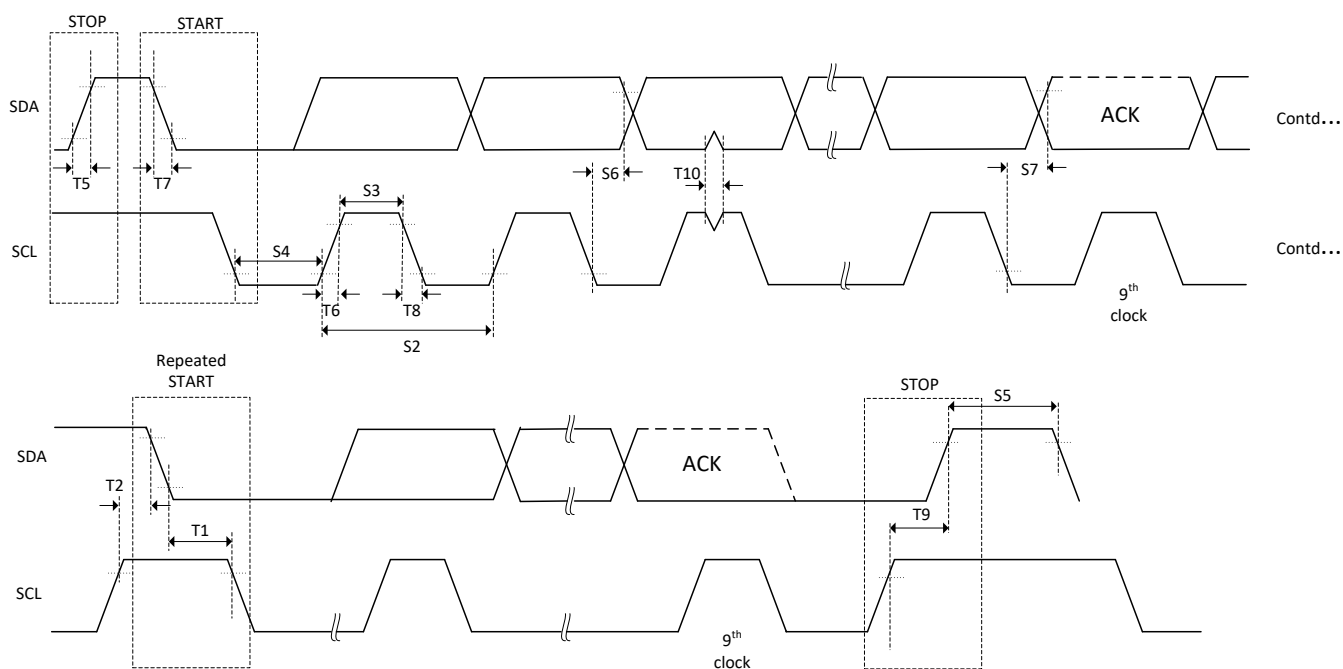
図 6-62. I2C タイミング図
