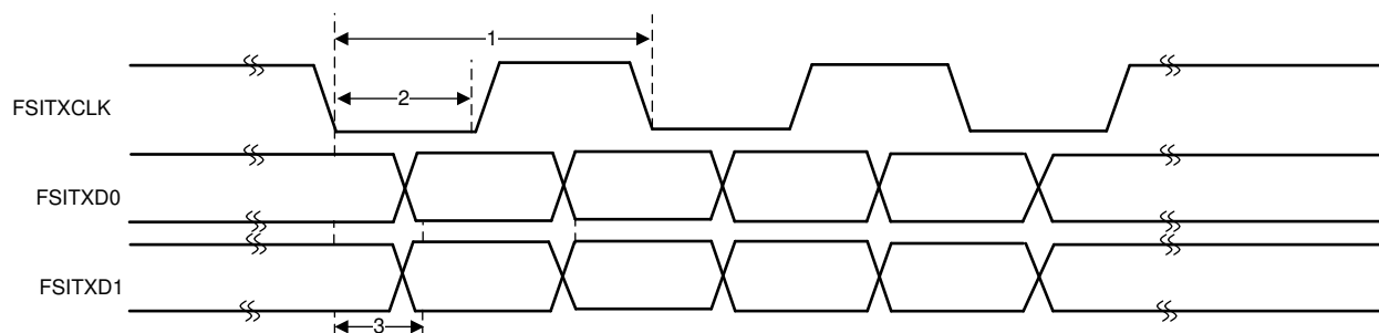
図 6-73. FSITX タイミング
