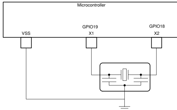
図 6-17. 外部共振子
