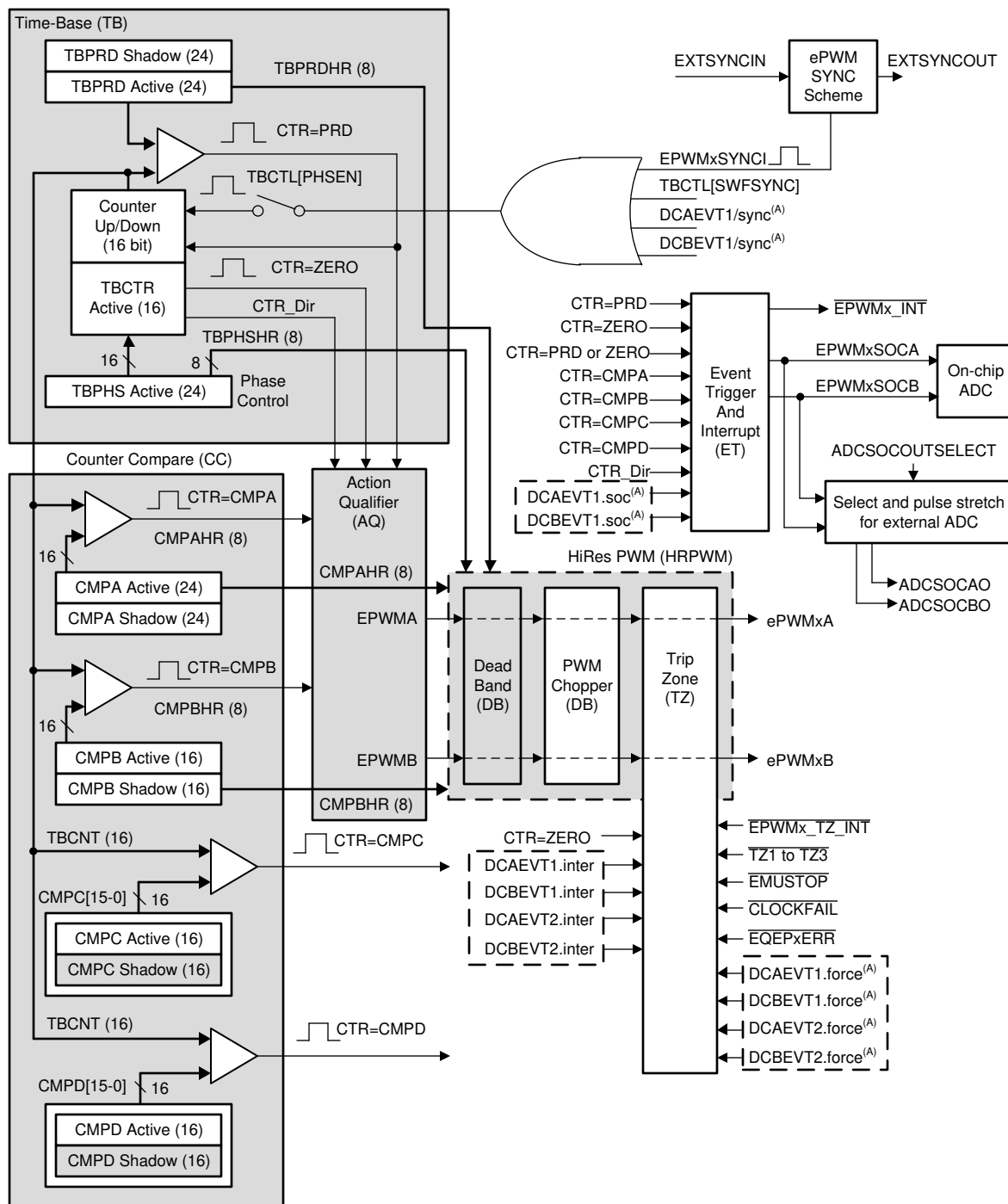
図 6-50. ePWM サブモジュールおよび重要な内部信号の相互接続
