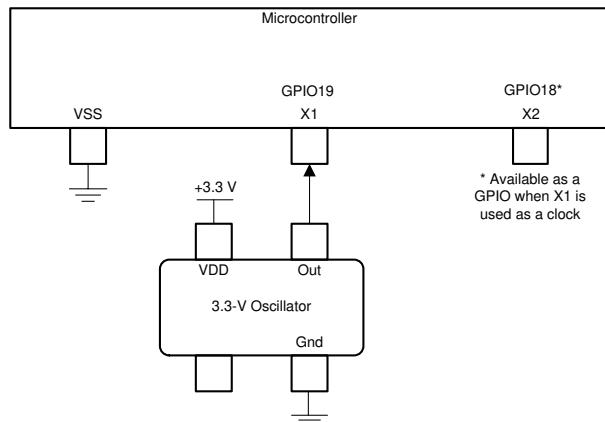
図 6-15. シングルエンド 3.3V 外部クロック
