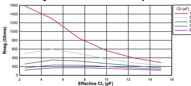
図 6-21. 20 MHz 時の負性抵抗変動
