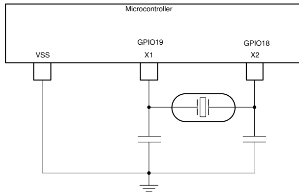
図 6-16. 外部水晶振動子
