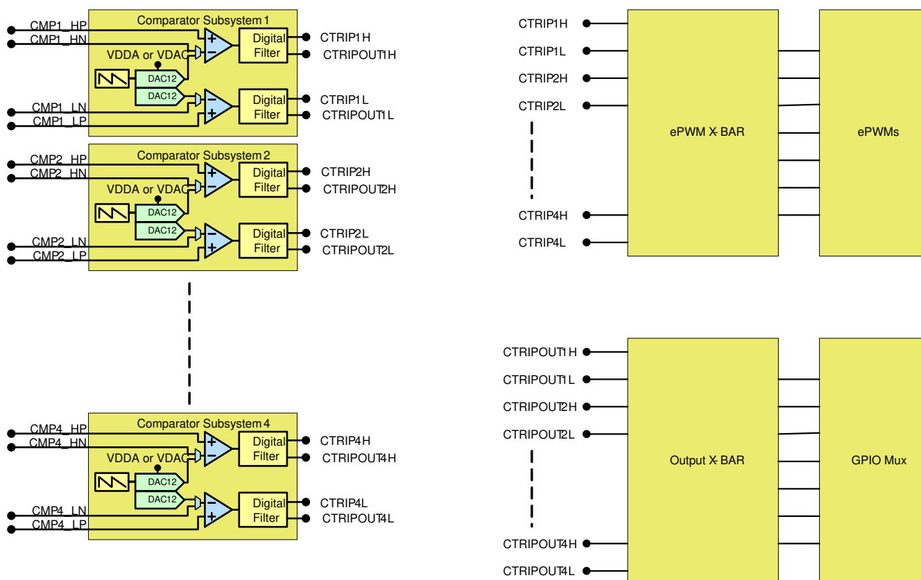
図 6-44. CMPSS の接続
