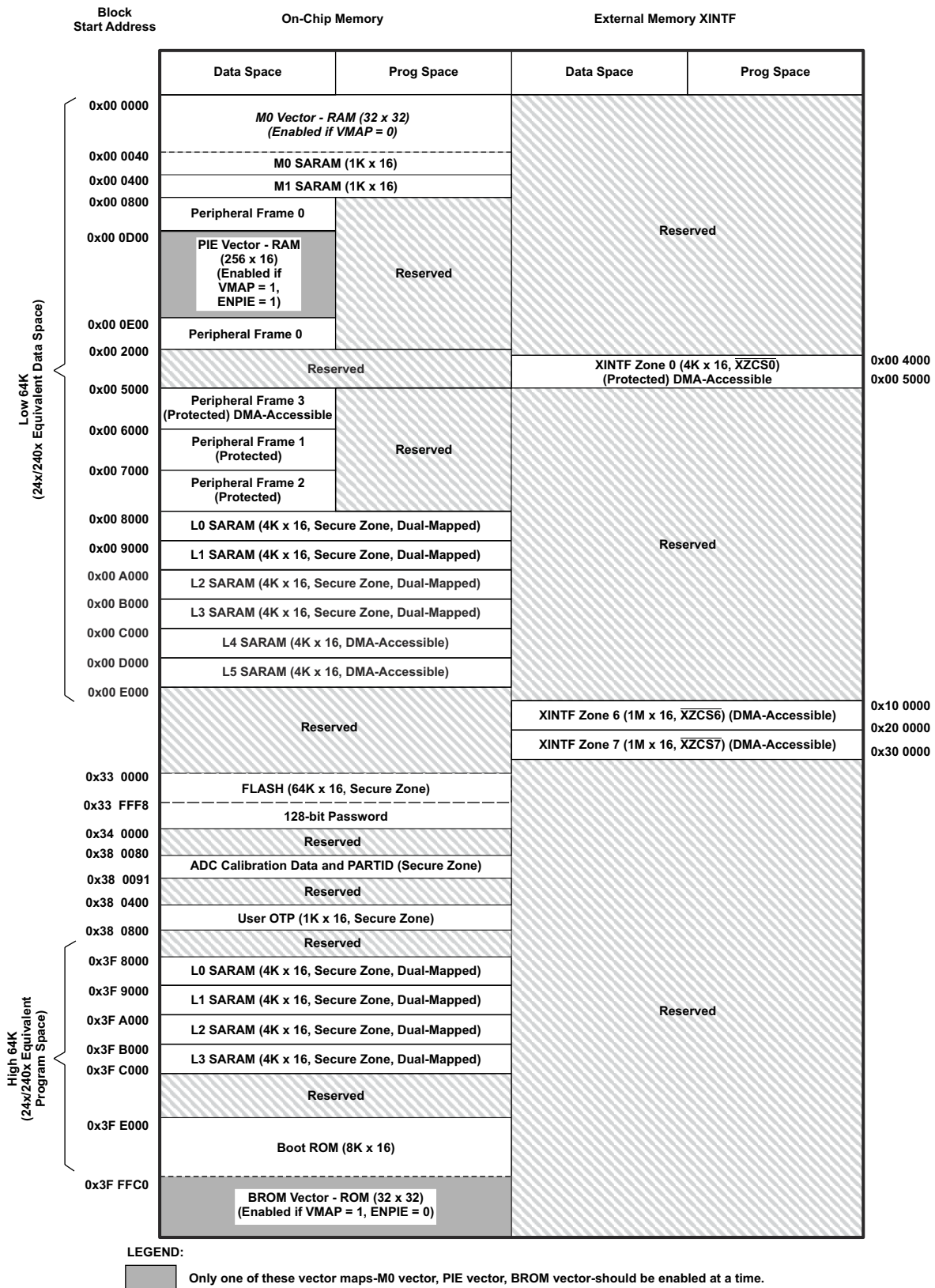
図 8-25. F28332、F28232 メモリ・マップ
