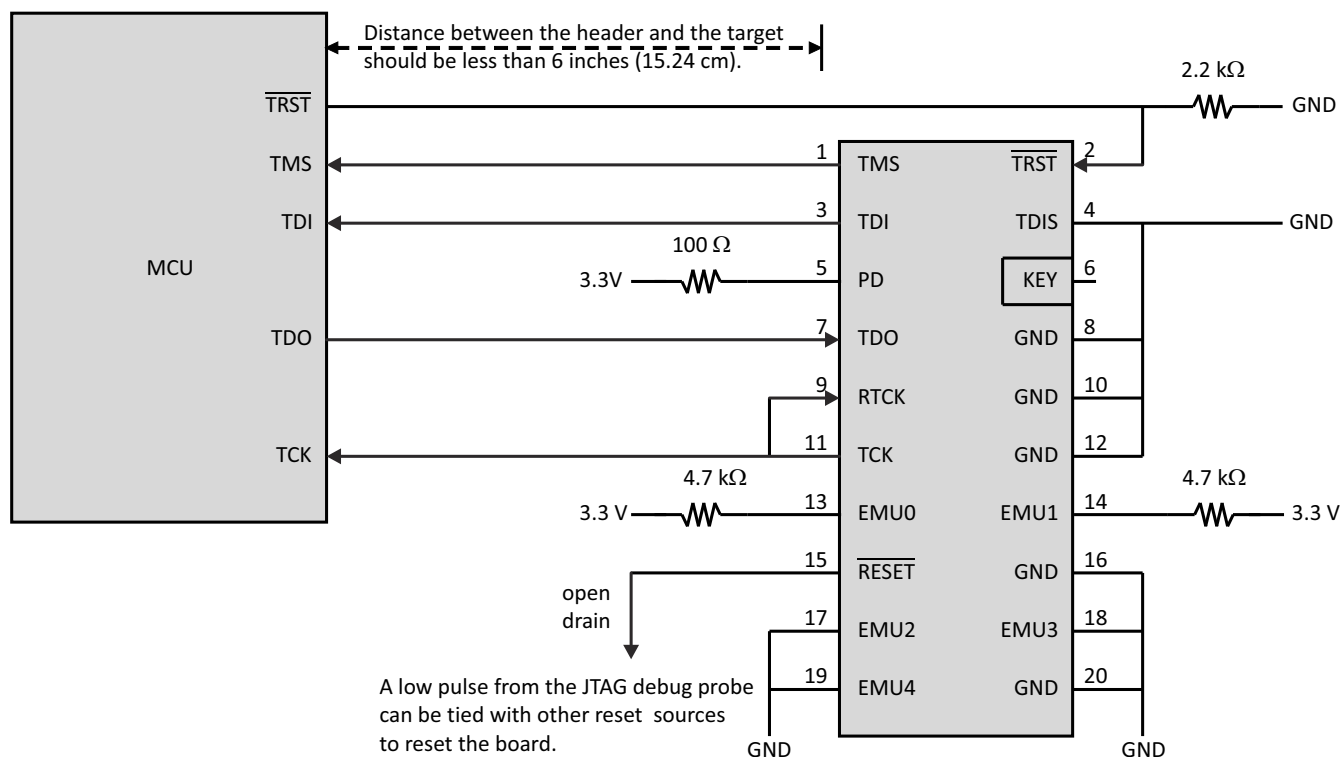
図 6-14. 20 ピン JTAG ヘッダーへの接続
