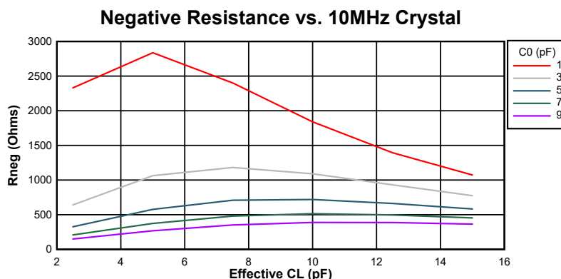
図 6-11. 10MHz 時の負性抵抗変動
