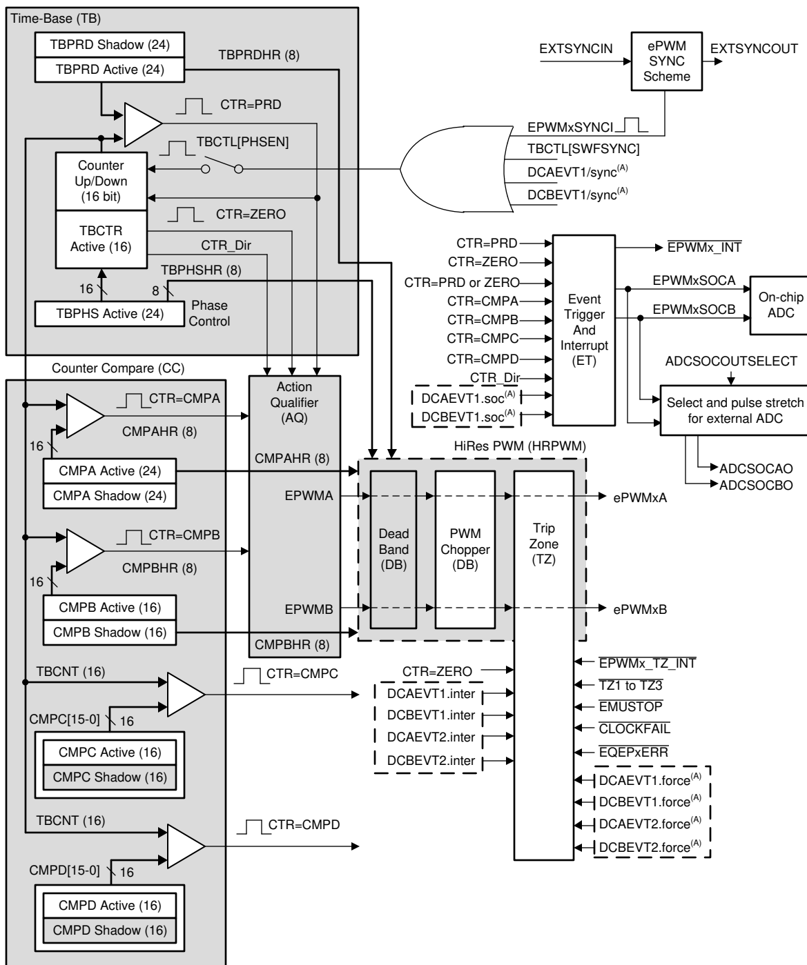
図 7-57. ePWM サブモジュールおよび重要な内部信号の相互接続
