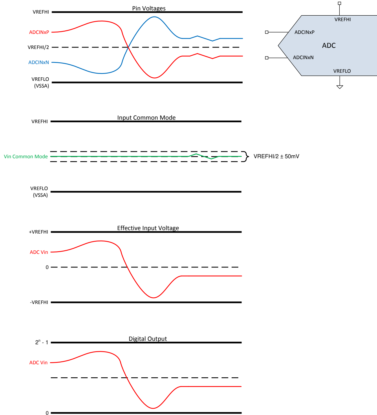
図 7-35. 差動信号モード
