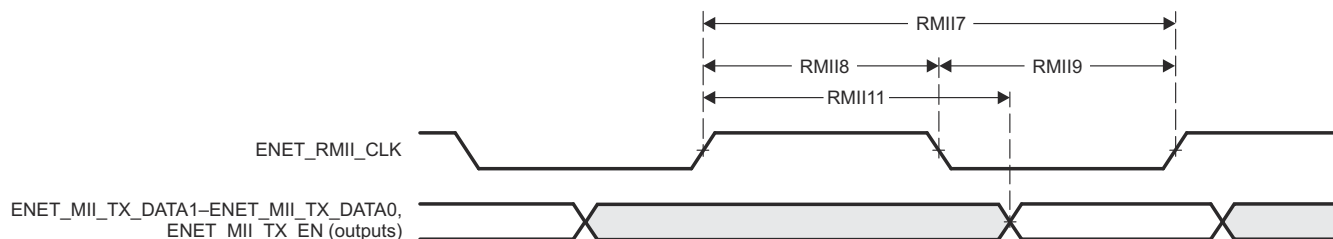
図 7-103. 送信インターフェースのタイミング (RMII 動作)
