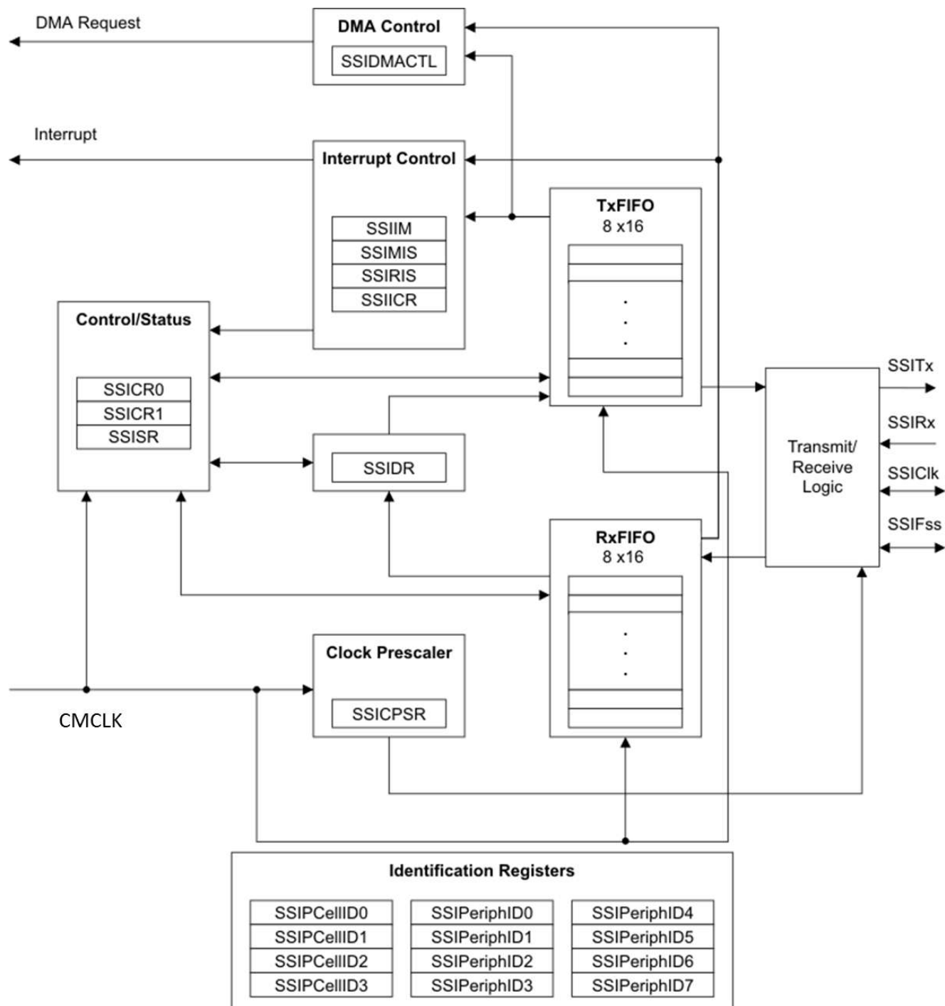
図 7-106. SSI のブロック図
