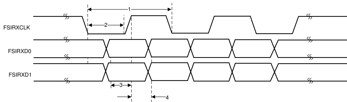
図 7-71. FSIRX タイミング
