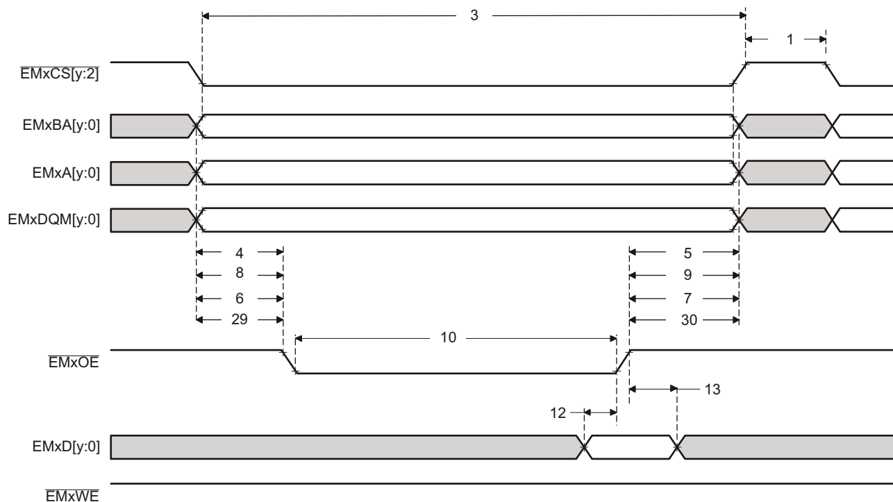
図 7-26. 非同期メモリ読み取りタイミング
