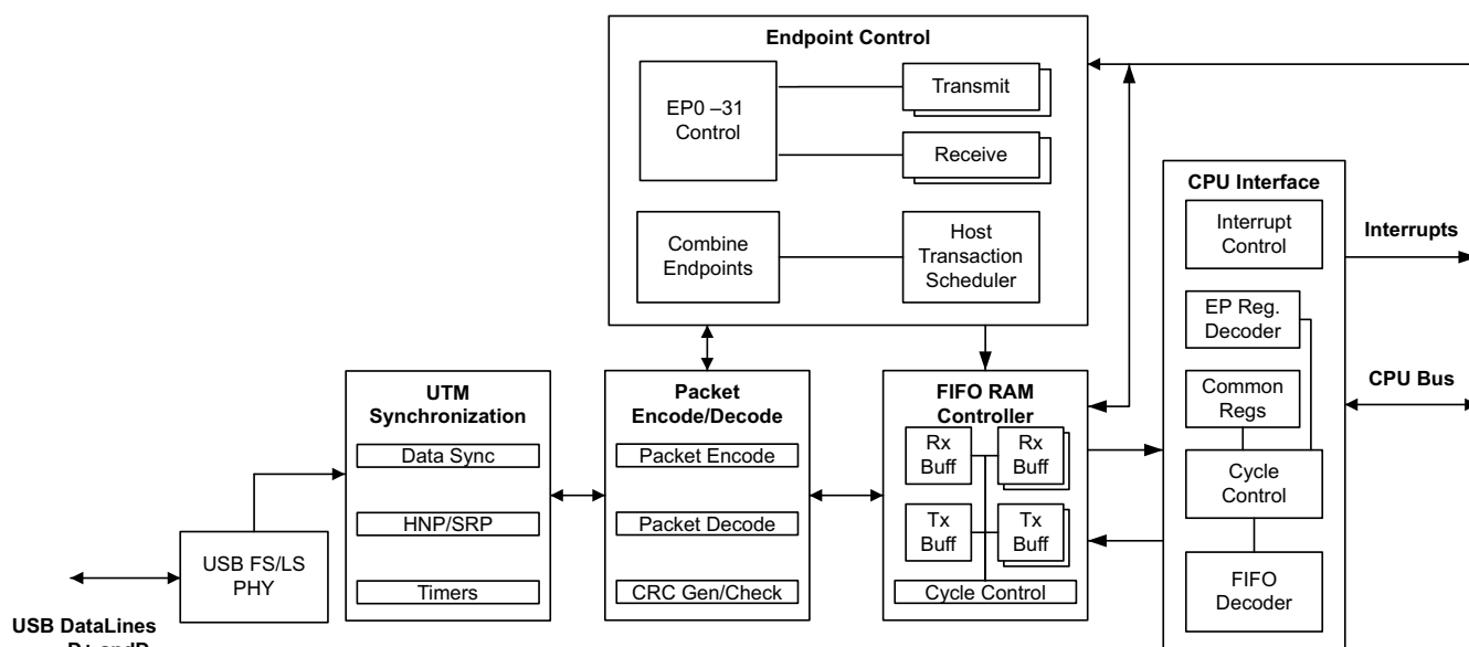
図 7-95. USB ブロック図
