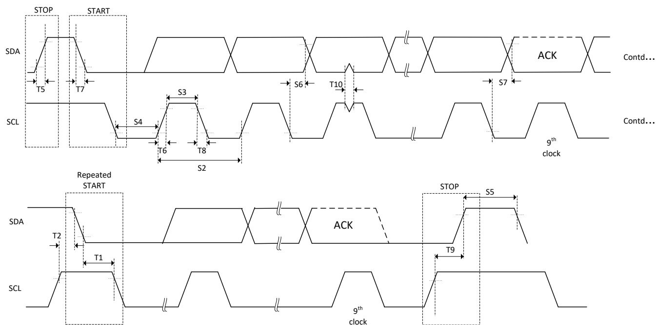
図 7-74. I2C のタイミング図
