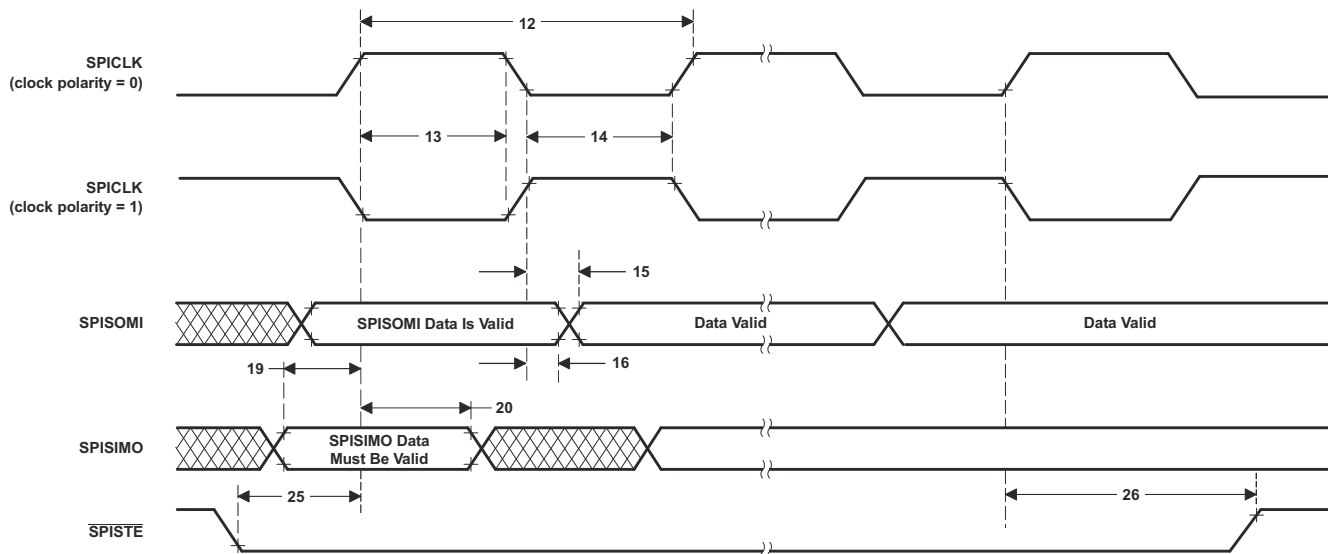
図 7-88. SPI スレーブ・モードの外部タイミング (クロック位相=1)
