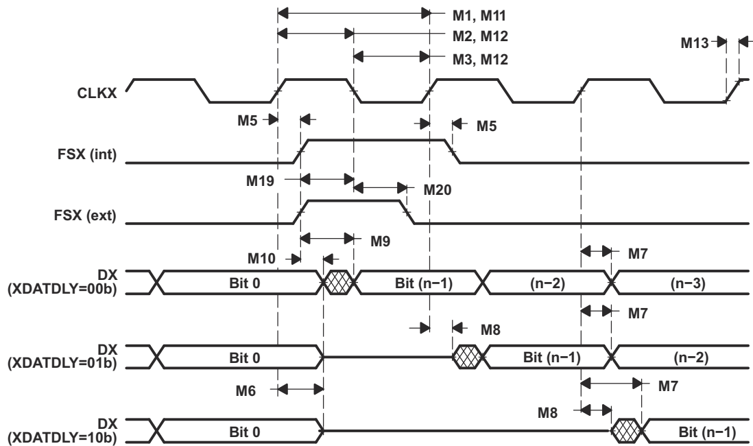
図 7-77. McBSP 送信タイミング
