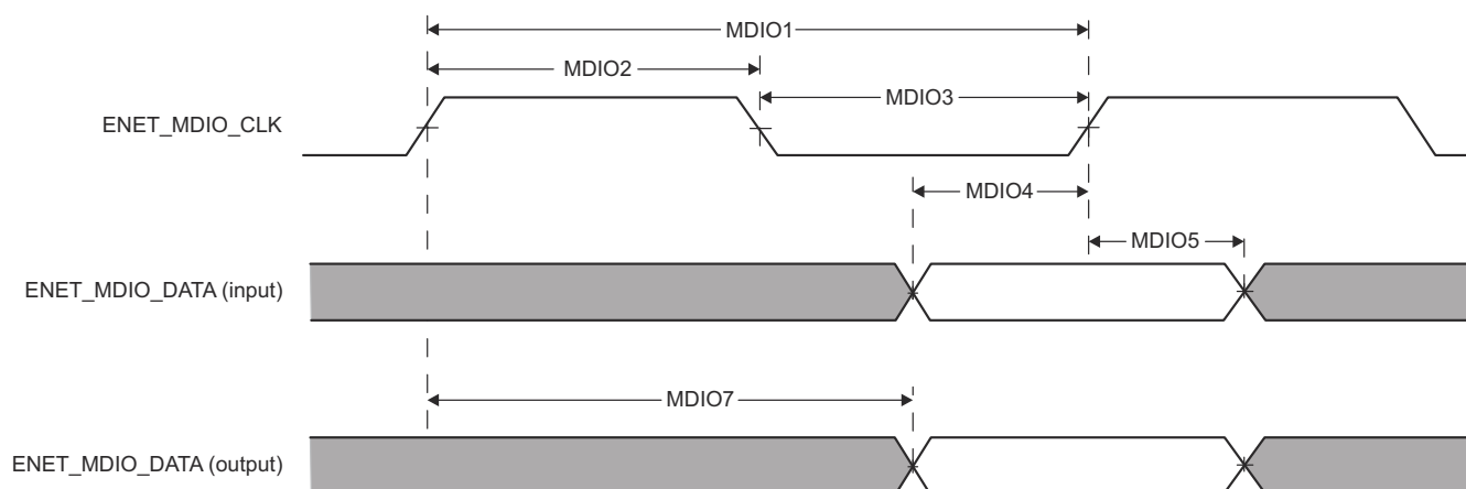
図 7-101. MDIO のタイミング図
