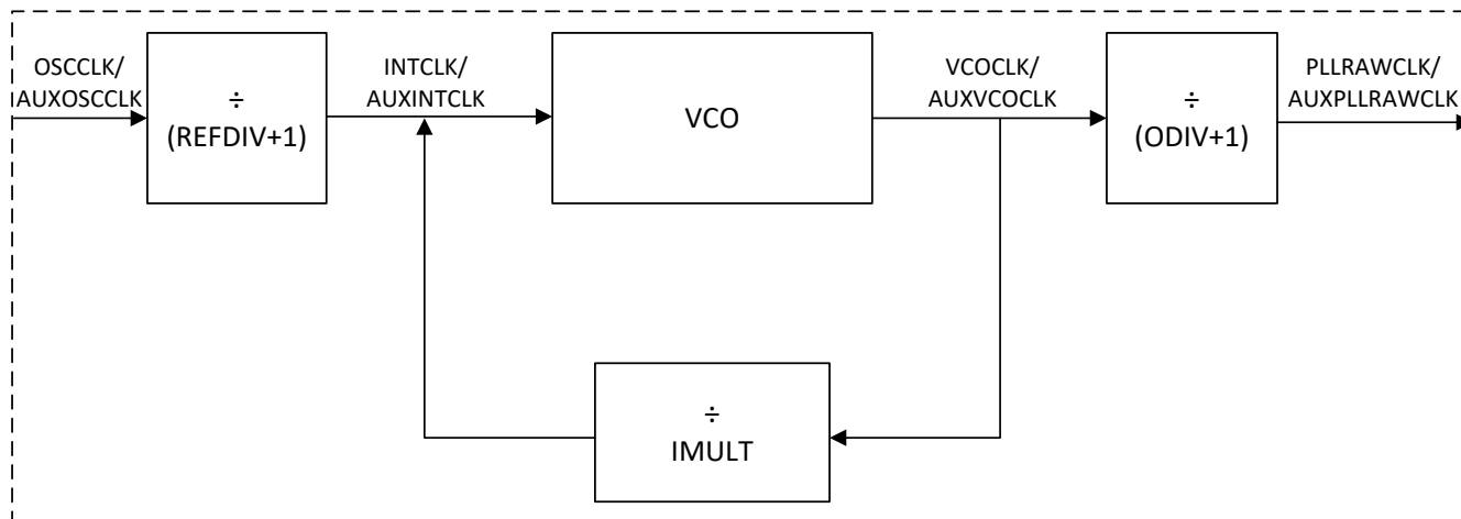
図 7-10. SYSPLL / AUXPLL
