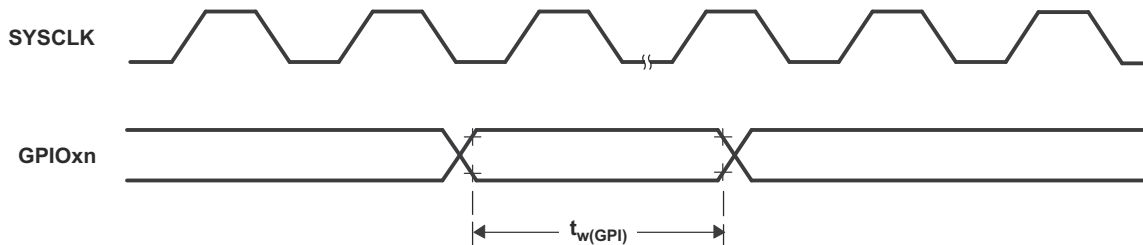
図 7-21. 汎用入力タイミグ
