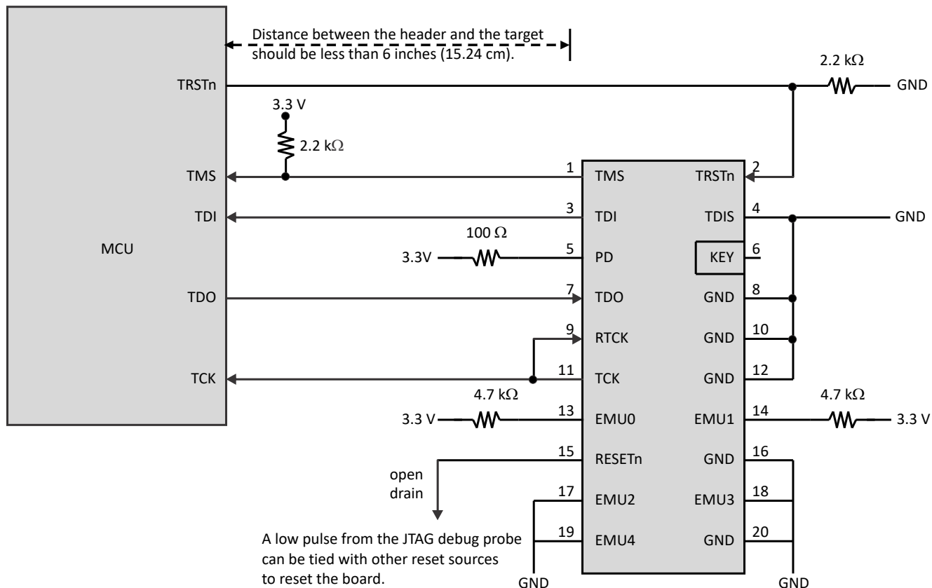
図 7-17. 20 ピン JTAG ヘッダーへの接続
