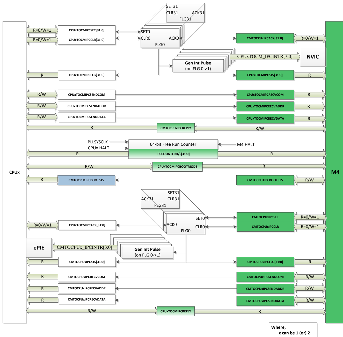
図 8-7. CPUx_to_CM IPC モジュール
