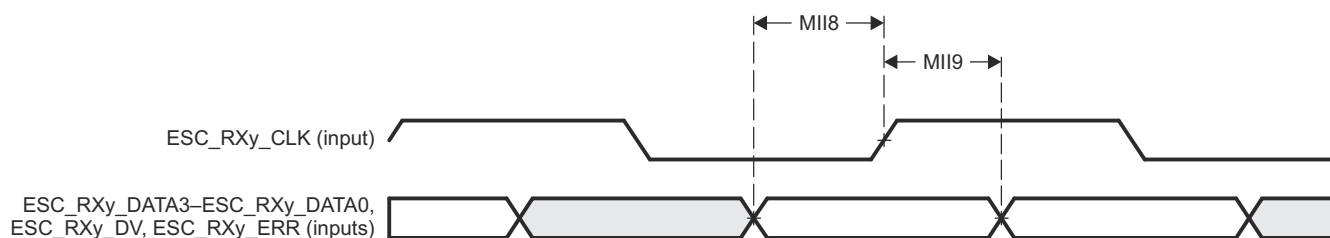
図 7-93. EtherCAT 受信インターフェースのタイミング (MII 動作)
