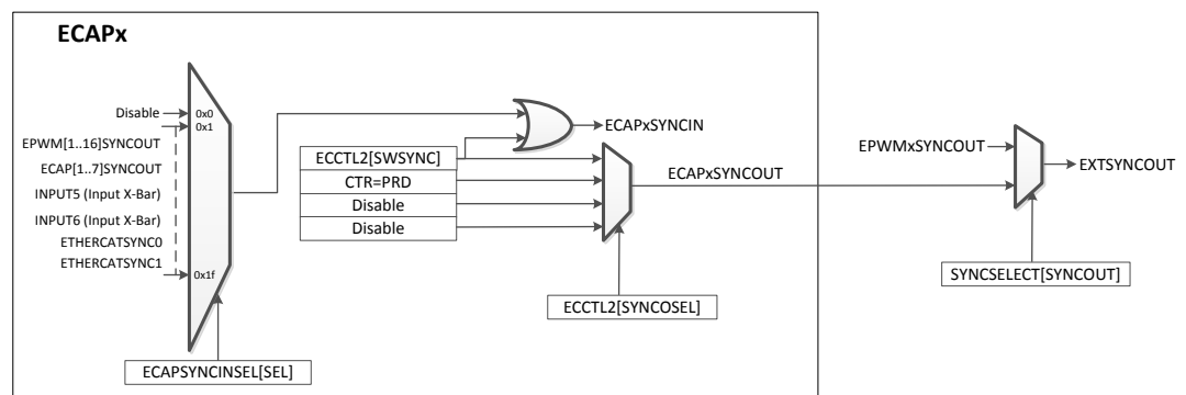
図 7-54. eCAPsynchronization 方式
