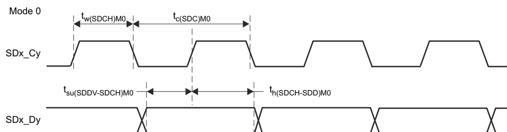
図 7-64. SDFM タイミング図 - モード 0
