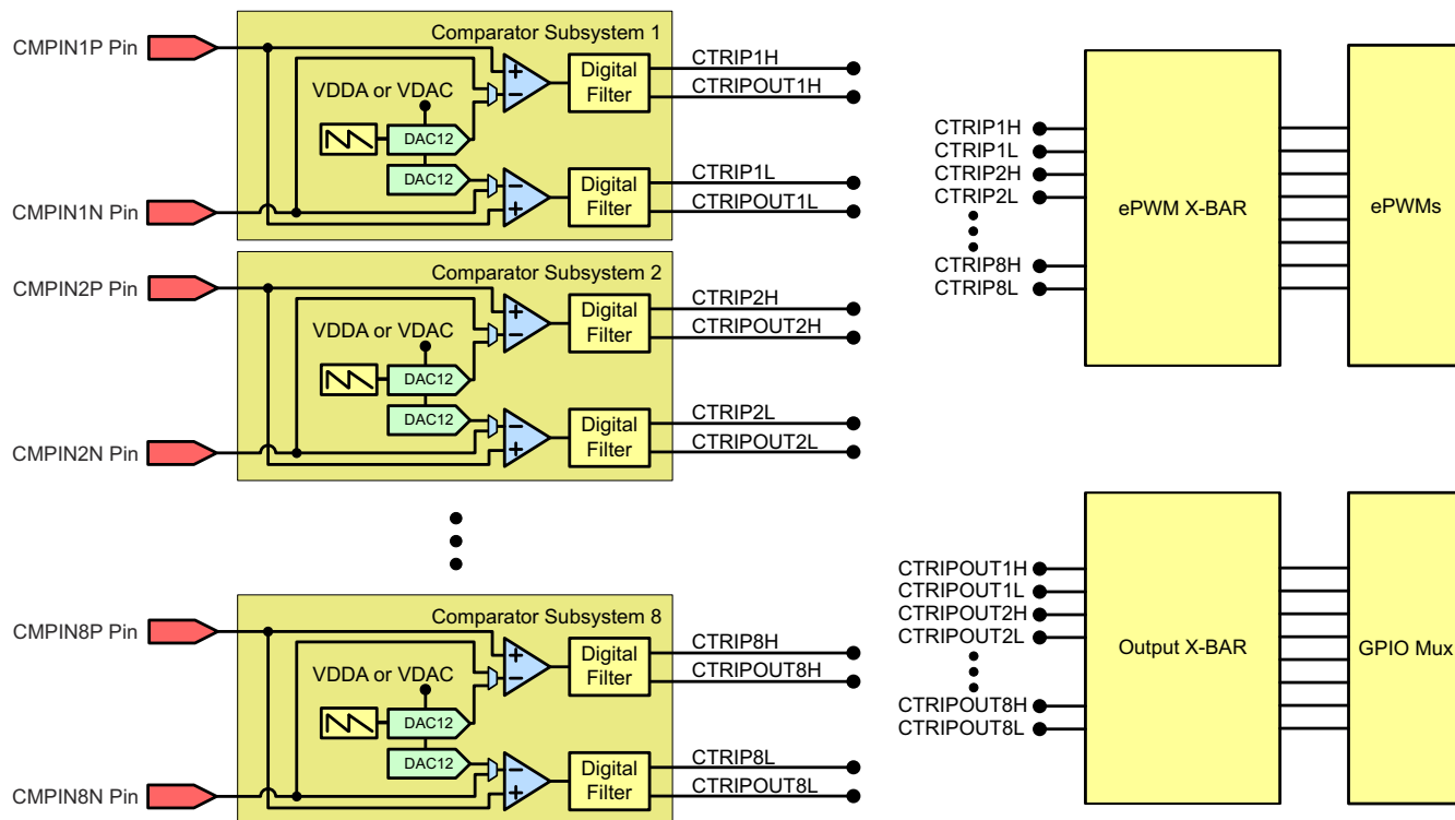
図 7-42. CMPSS 接続 (337 ボール ZWT および 176 ピン PTP)
