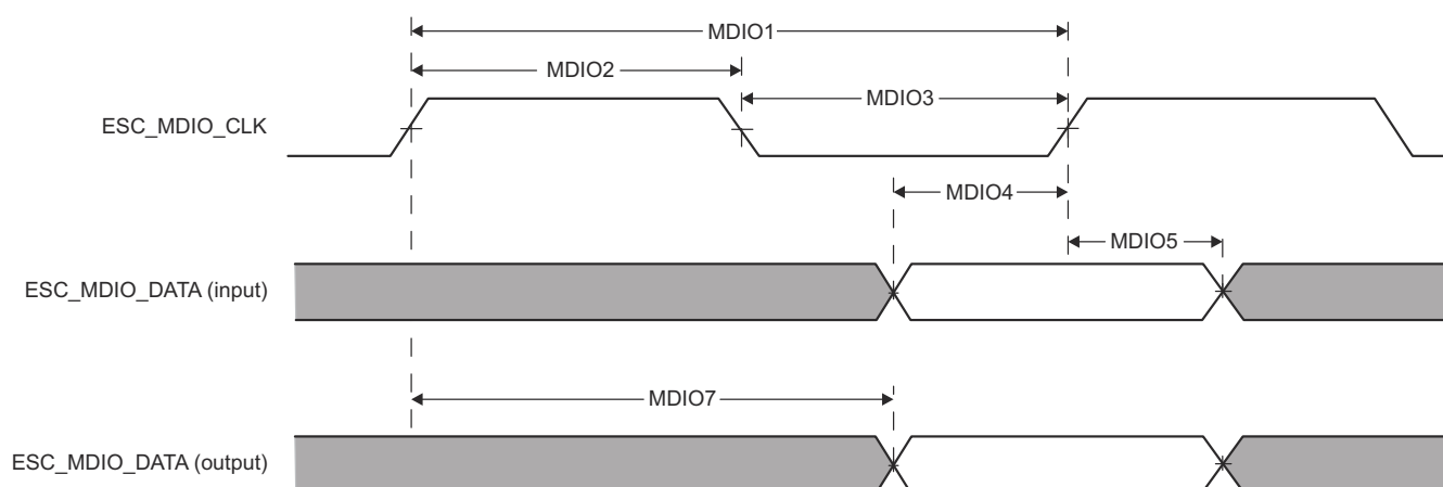
図 7-94. EtherCAT MDIO のタイミング図
