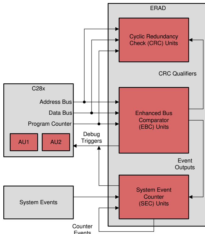
図 8-2. ERAD の概要
