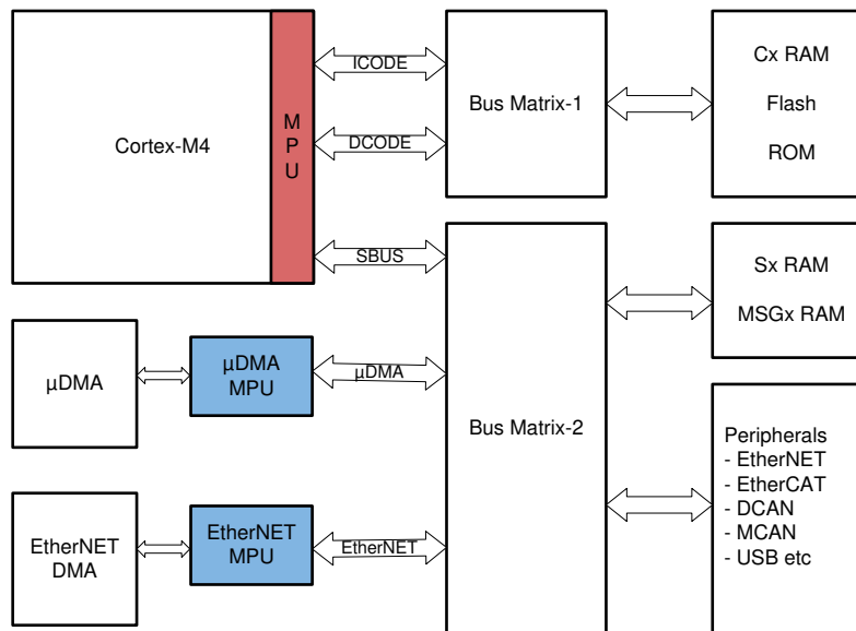
図 8-13. CM のブロック図
