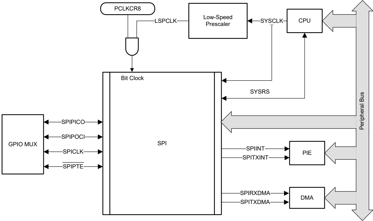
図 6-73. SPI CPU インターフェイス
