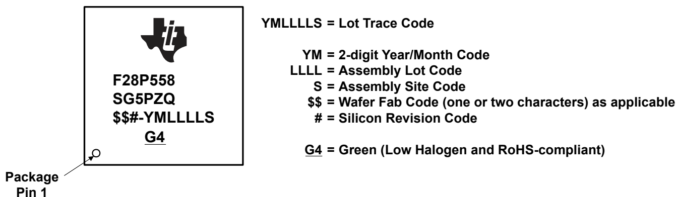
図 9-4. PZ パッケージのパッケージ マーキング – 車載
