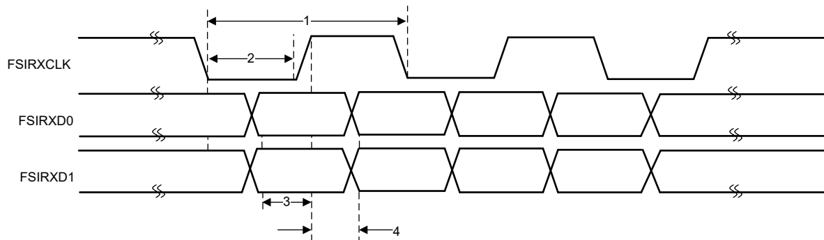
図 6-84. FSIRX タイミング
