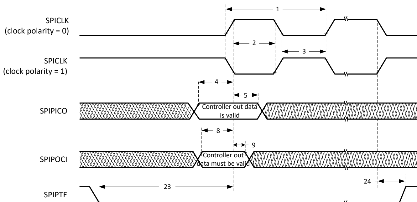
図 6-74. SPI コントローラ・モードの外部タイミング (クロック位相 = 0)
