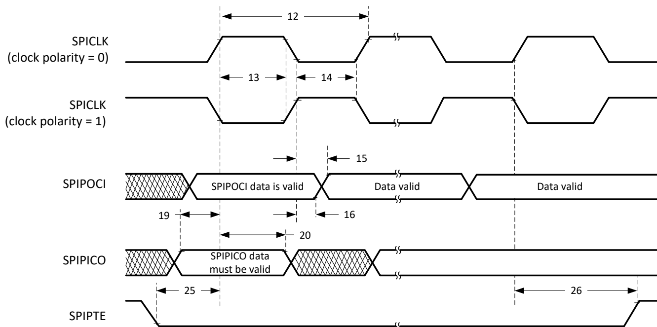
図 6-77. SPI ペリフェラル・モードの外部タイミング (クロック位相 = 1)
