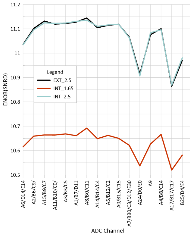
図 6-44. 49 ボール YAF のチャンネルごとの ENOB
