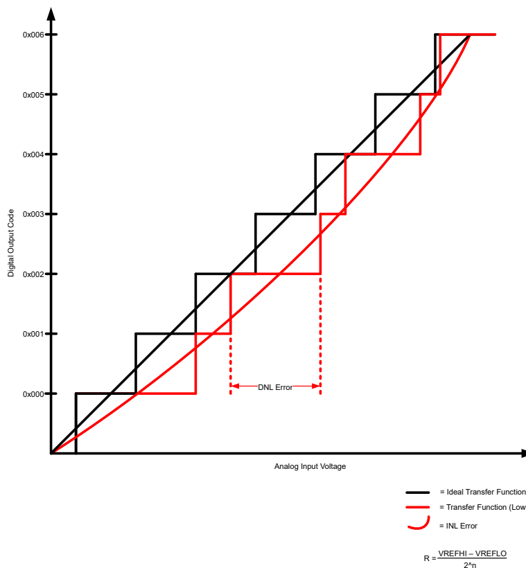
図 6-39. ADC の INL と DNL
