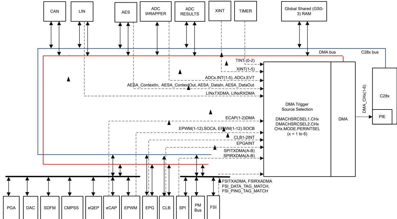
図 7-3. DMA のブロック図
