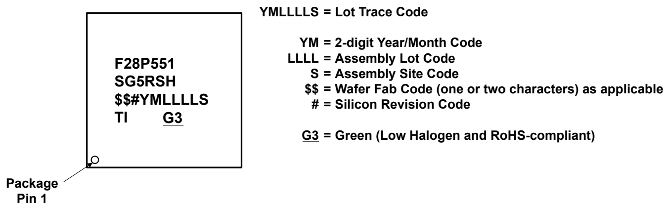
図 9-11. RSH パッケージのパッケージ マーキング – 車載以外
