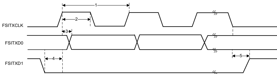
図 6-85. FSITX SPI 信号モードのタイミング
