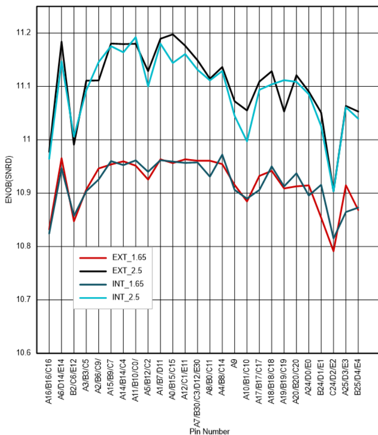
図 6-42. 64 ピン PM のチャンネルごとの ENOB
