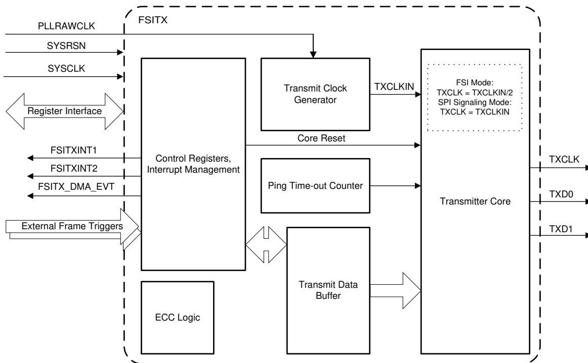
図 6-80. FSITX のブロック図
