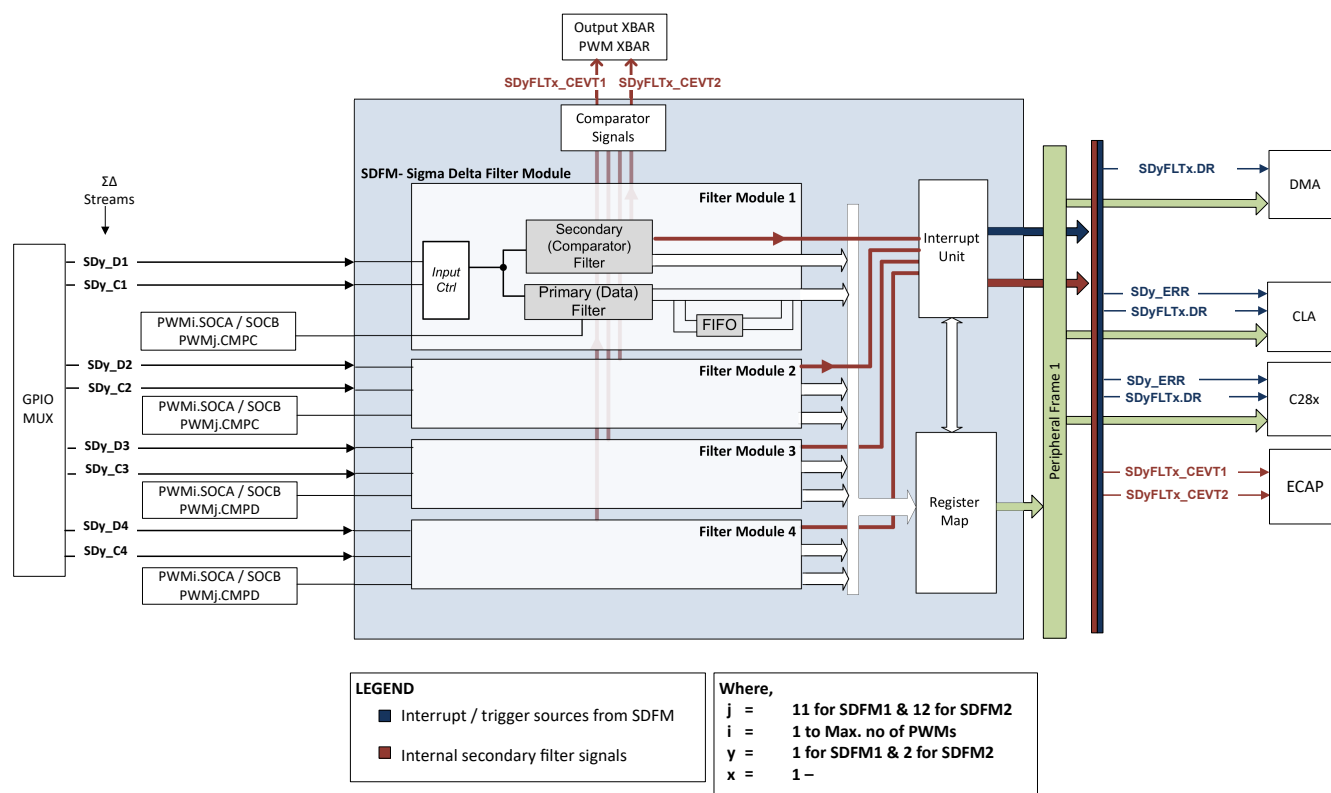
図 6-66. シグマ デルタ フィルタ モジュール (SDFM) のブロック図
