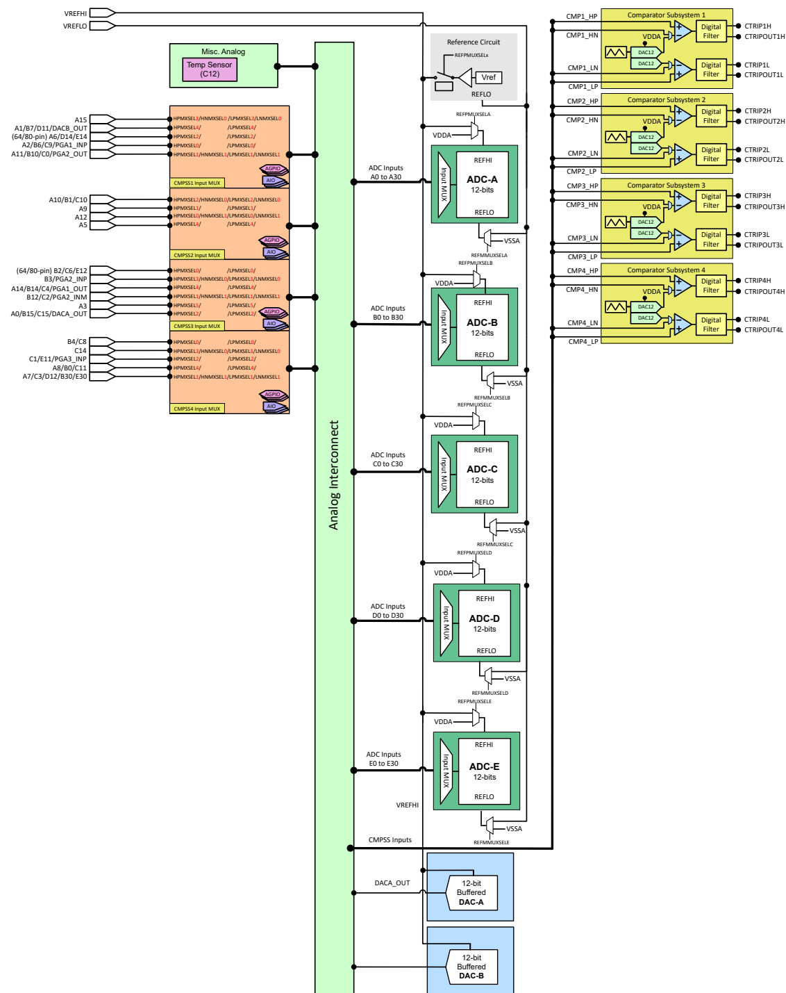
図 6-34. アナログ サブシステムのブロック図 (80/64/56 ピン パッケージ)
