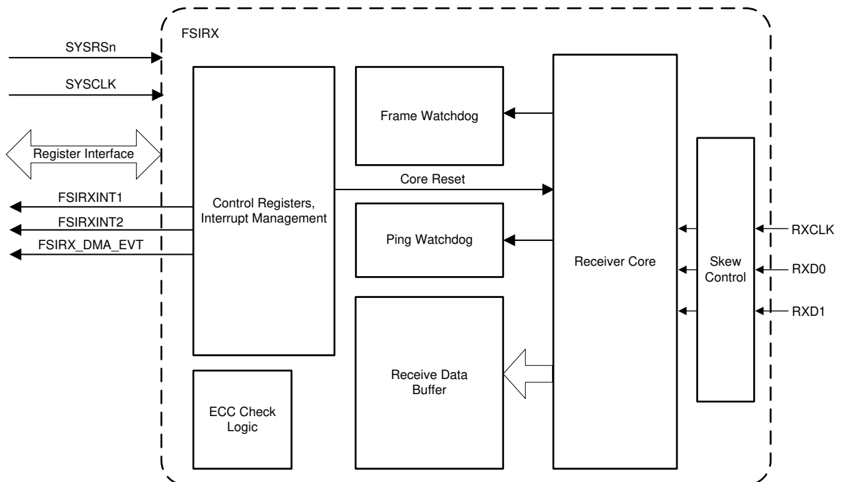
図 6-83. FSIRX のブロック図
