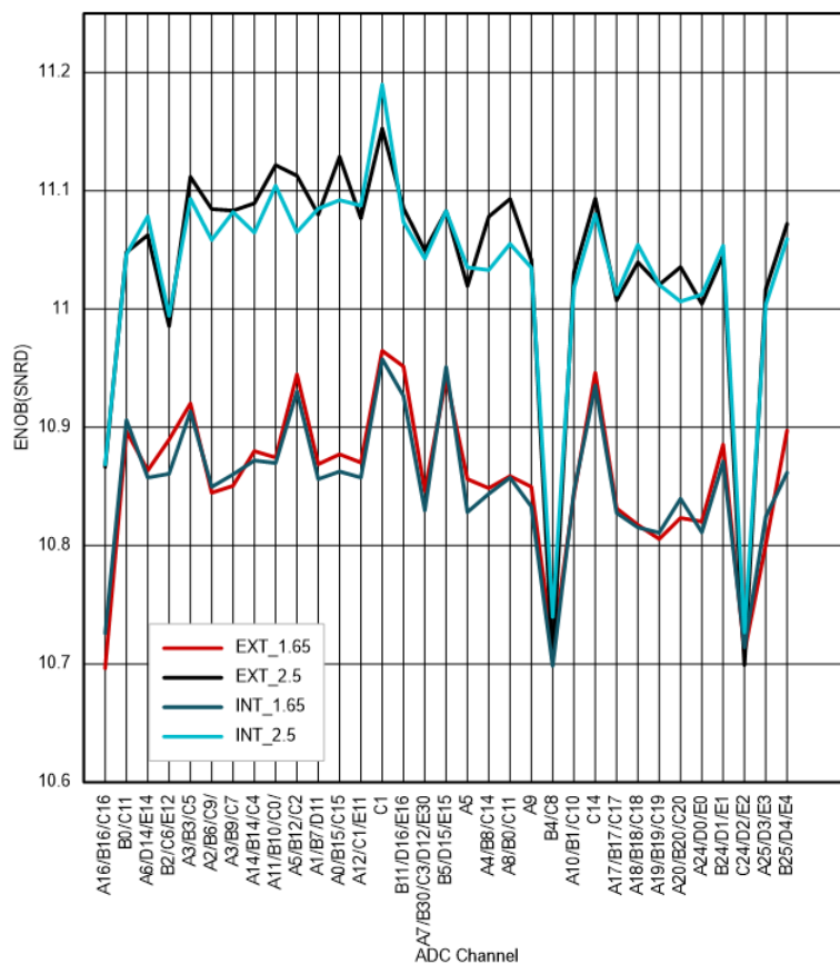
図 6-40. 100 ピン PZ のチャンネルごとの ENOB
