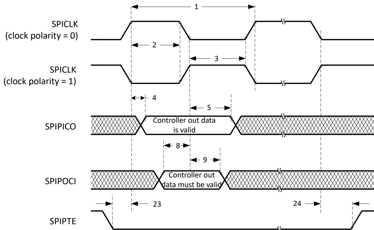
図 6-74. SPI コントローラ・モードの外部タイミング (クロック位相 = 0)
