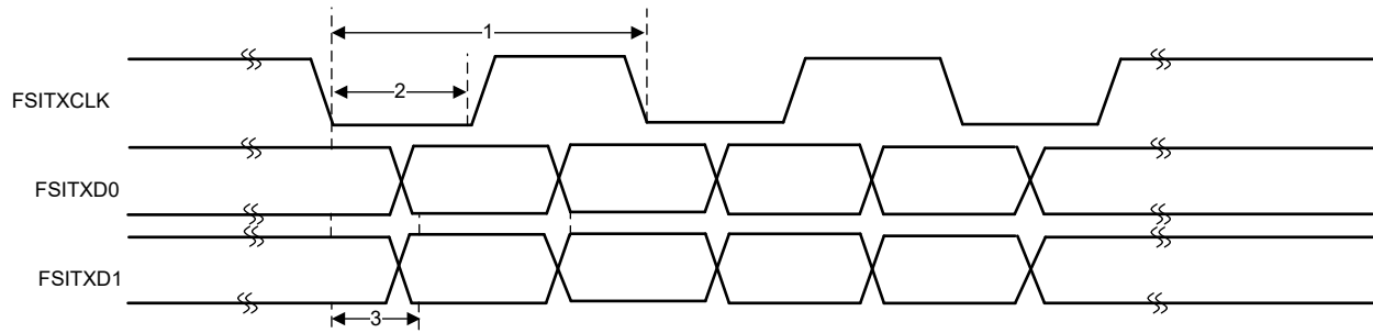
図 6-81. FSITX タイミング
