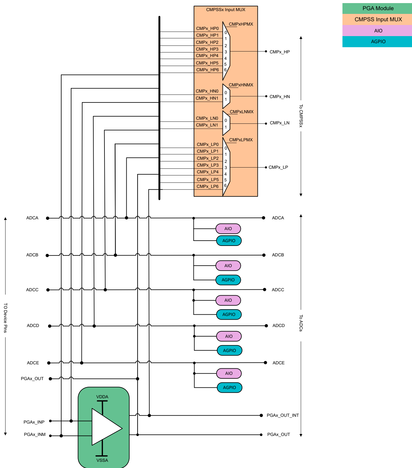
図 6-36. アナログ グループ接続
