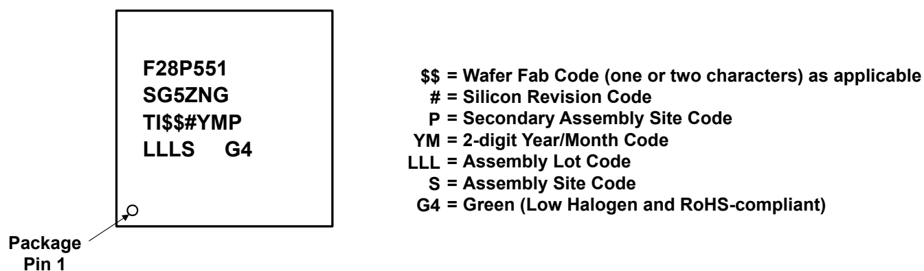
図 9-13. ZNG パッケージのパッケージ マーキング – 車載以外
