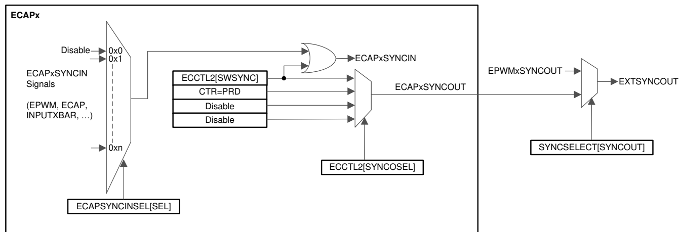
図 6-64. eCAP の同期方式
