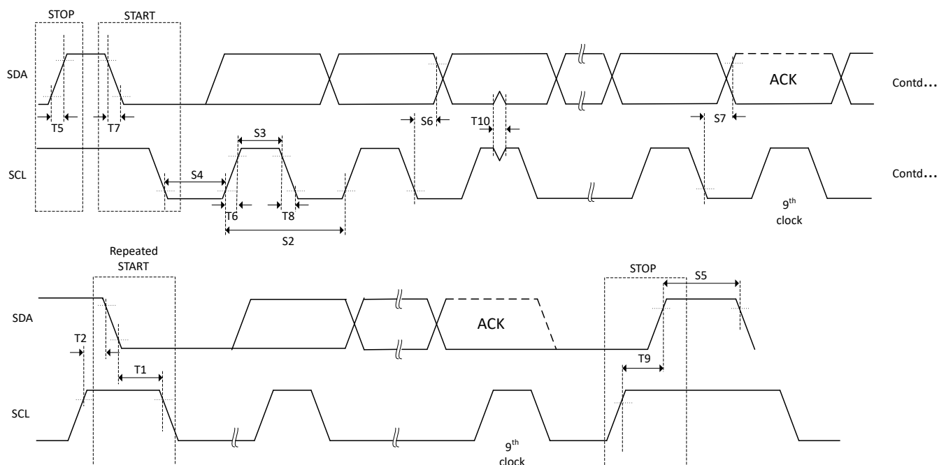
図 6-70. I2C のタイミング図
