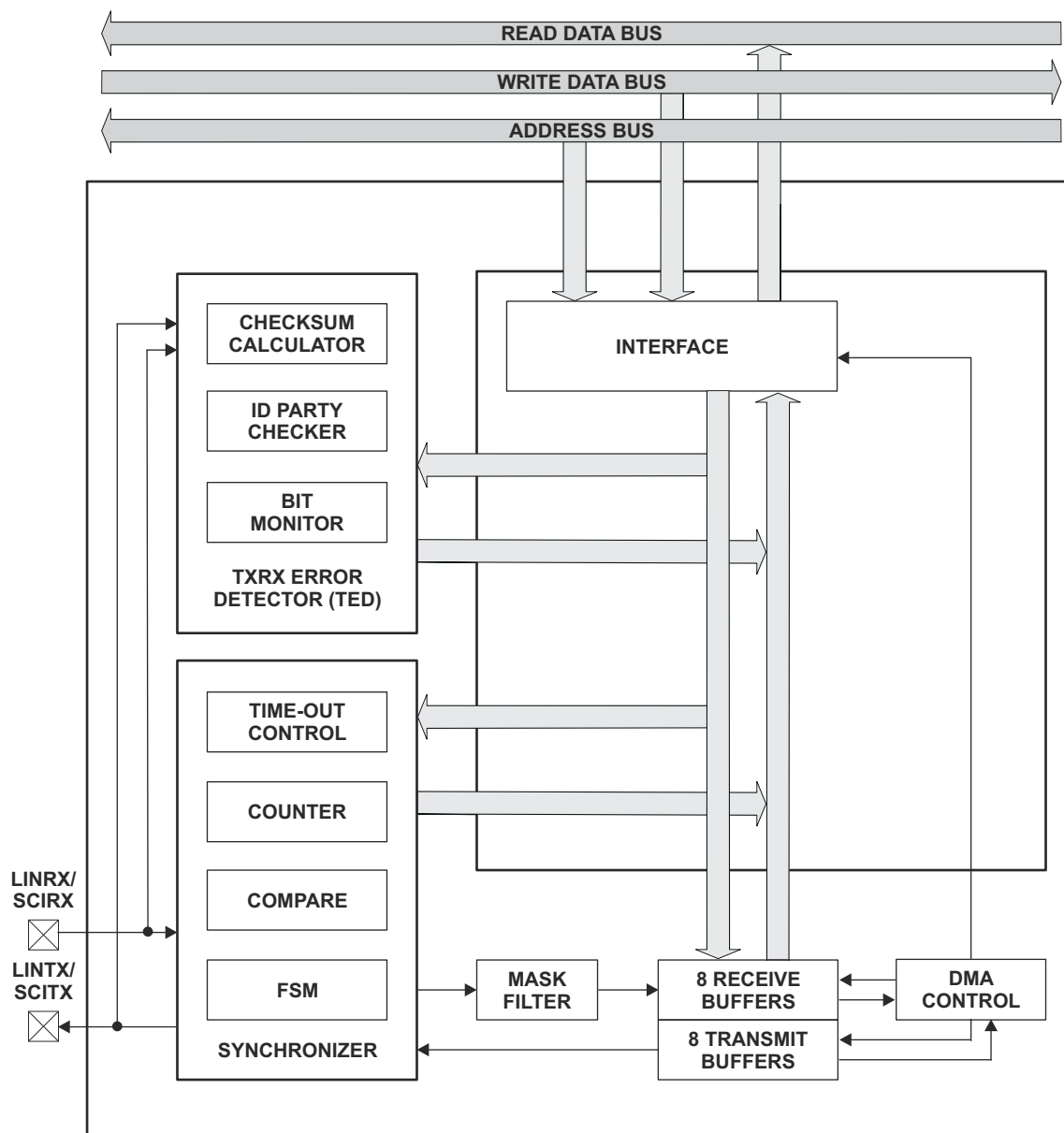
図 6-78. LIN のブロック図
