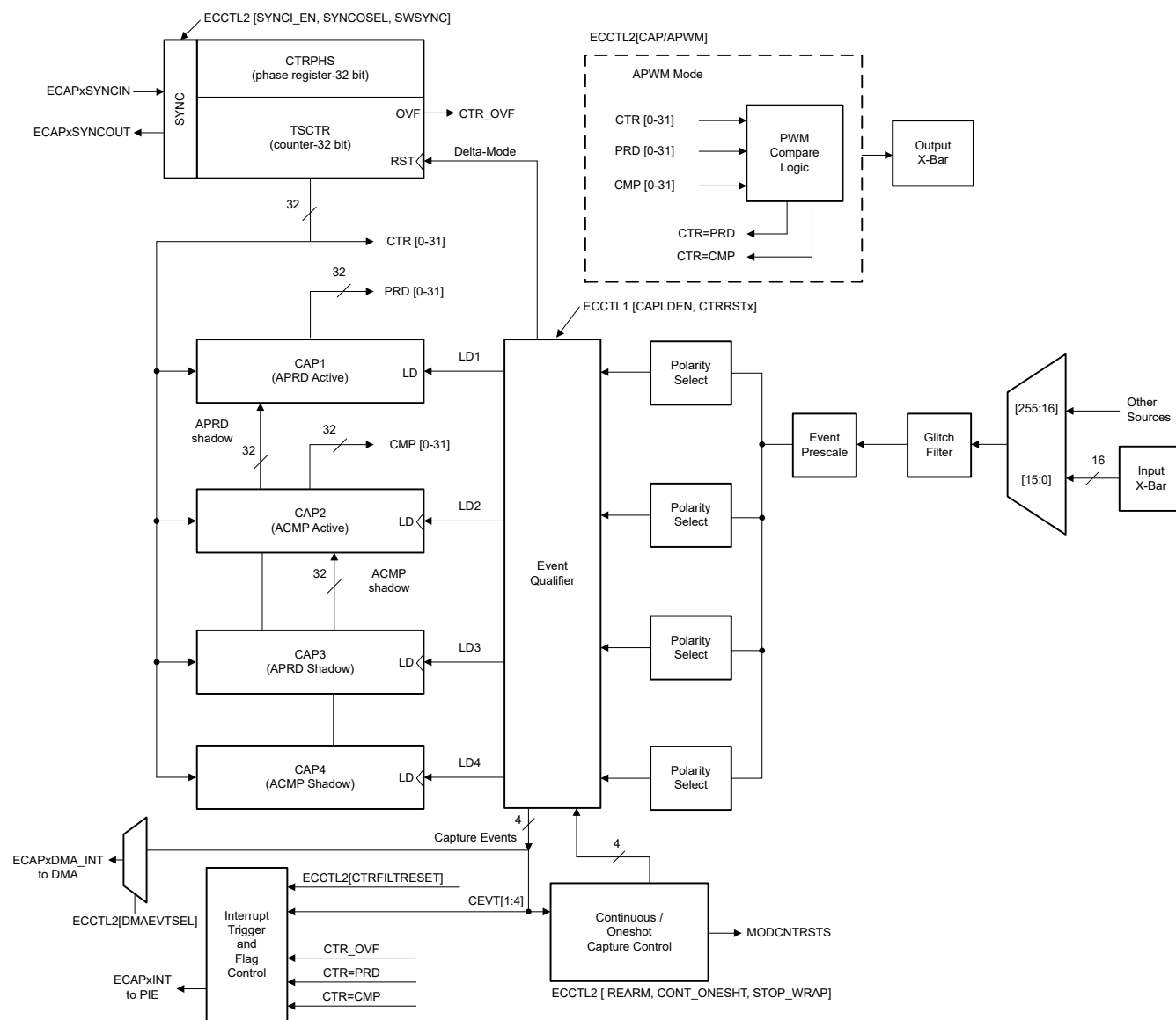
図 6-63. eCAP のブロック図
