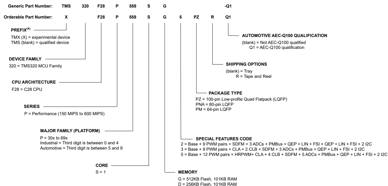
図 9-1. デバイスの命名規則 P558
