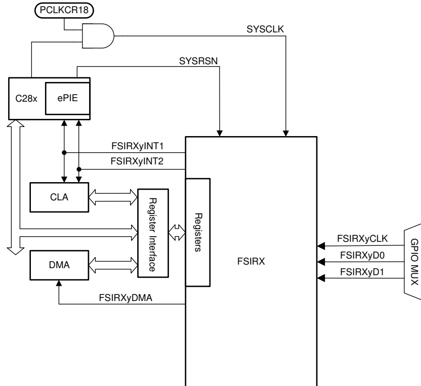
図 6-82. FSIRX CPU インターフェイス
