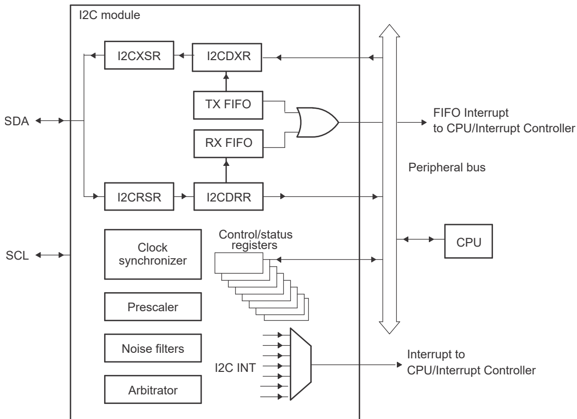
図 6-69. I2C ペリフェラル モジュール インターフェイス
