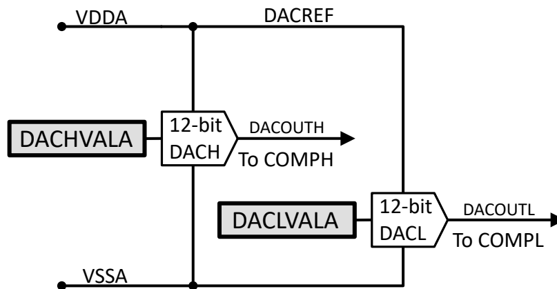
図 6-50. リファレンス DAC のブロック図
