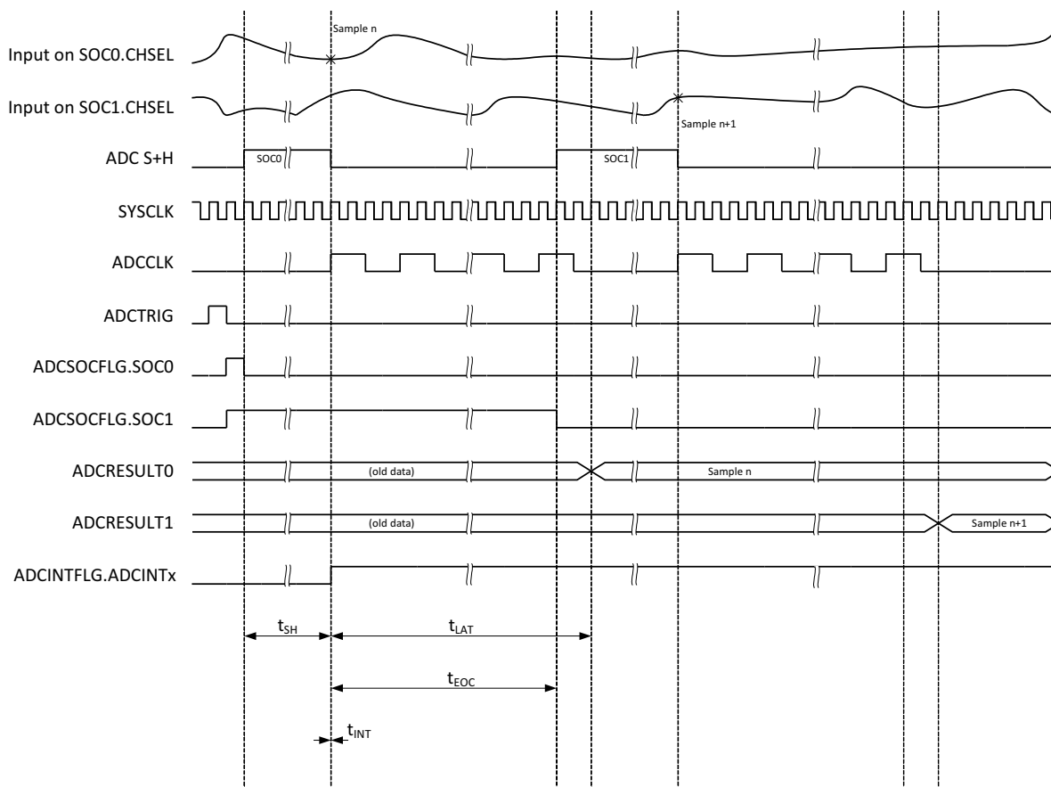
図 6-46. 12 ビット モードの Early 割り込みモードでの ADC タイミング
