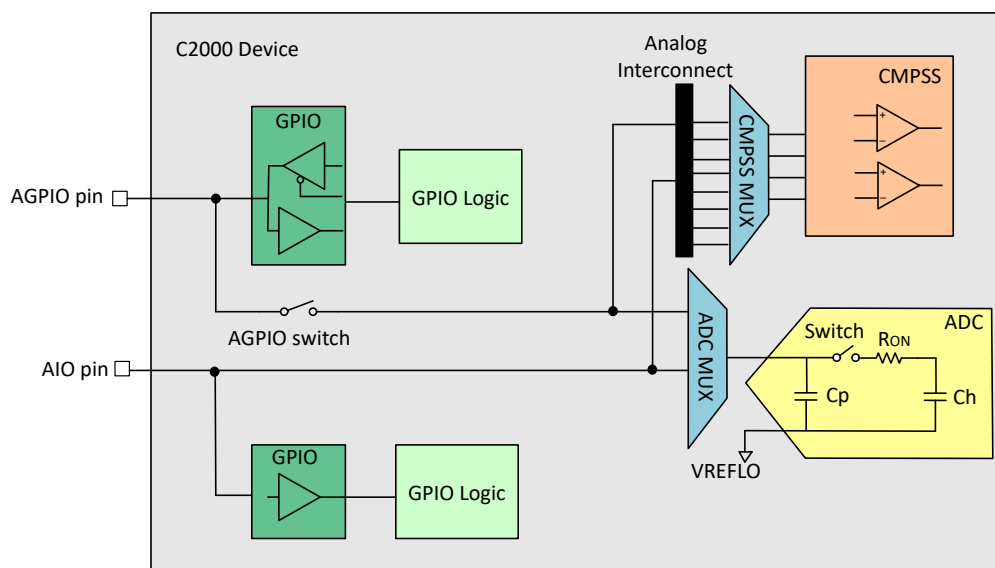
図 5-8. AGPIO を実装したアナログ サブシステムのブロック図
