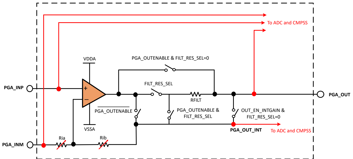
図 6-57. PGA のブロック図
