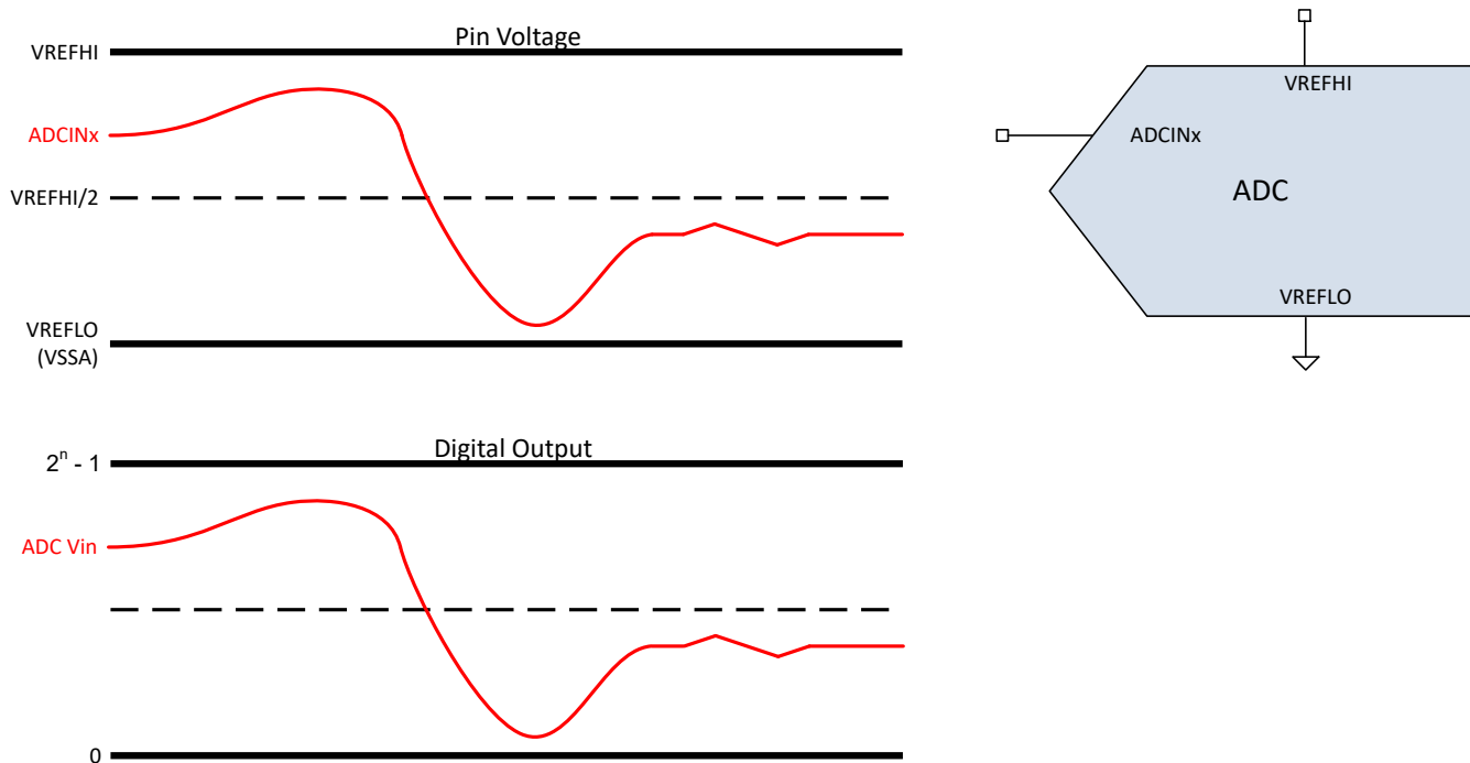
図 6-38. シングルエンド信号モード
