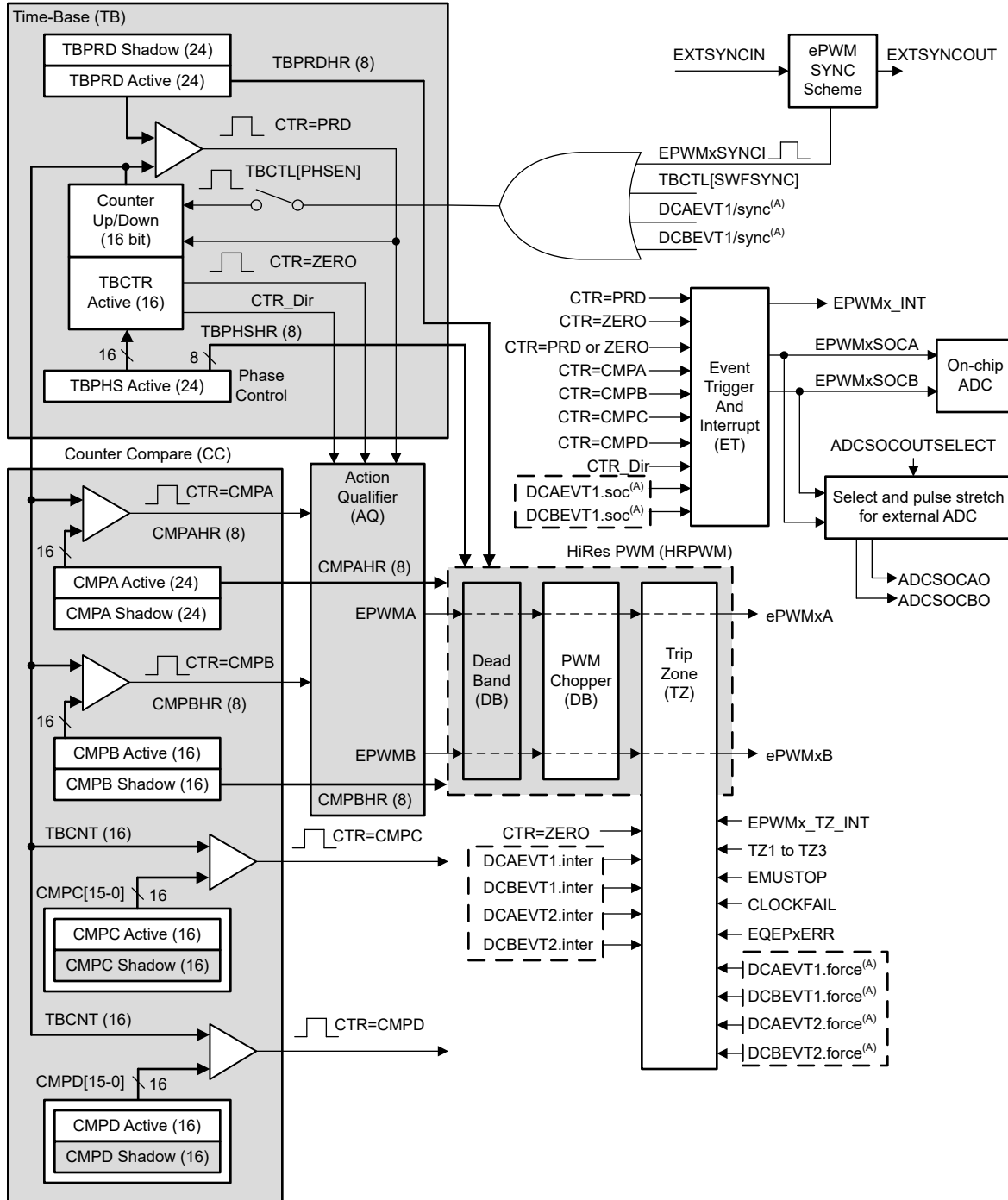
図 6-58. ePWM サブモジュールおよび重要な内部信号の相互接続
