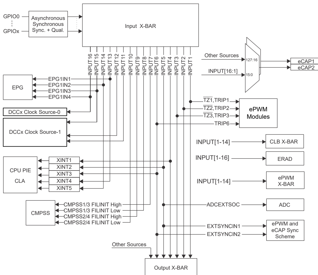
図 5-9. 入力クロスバー
