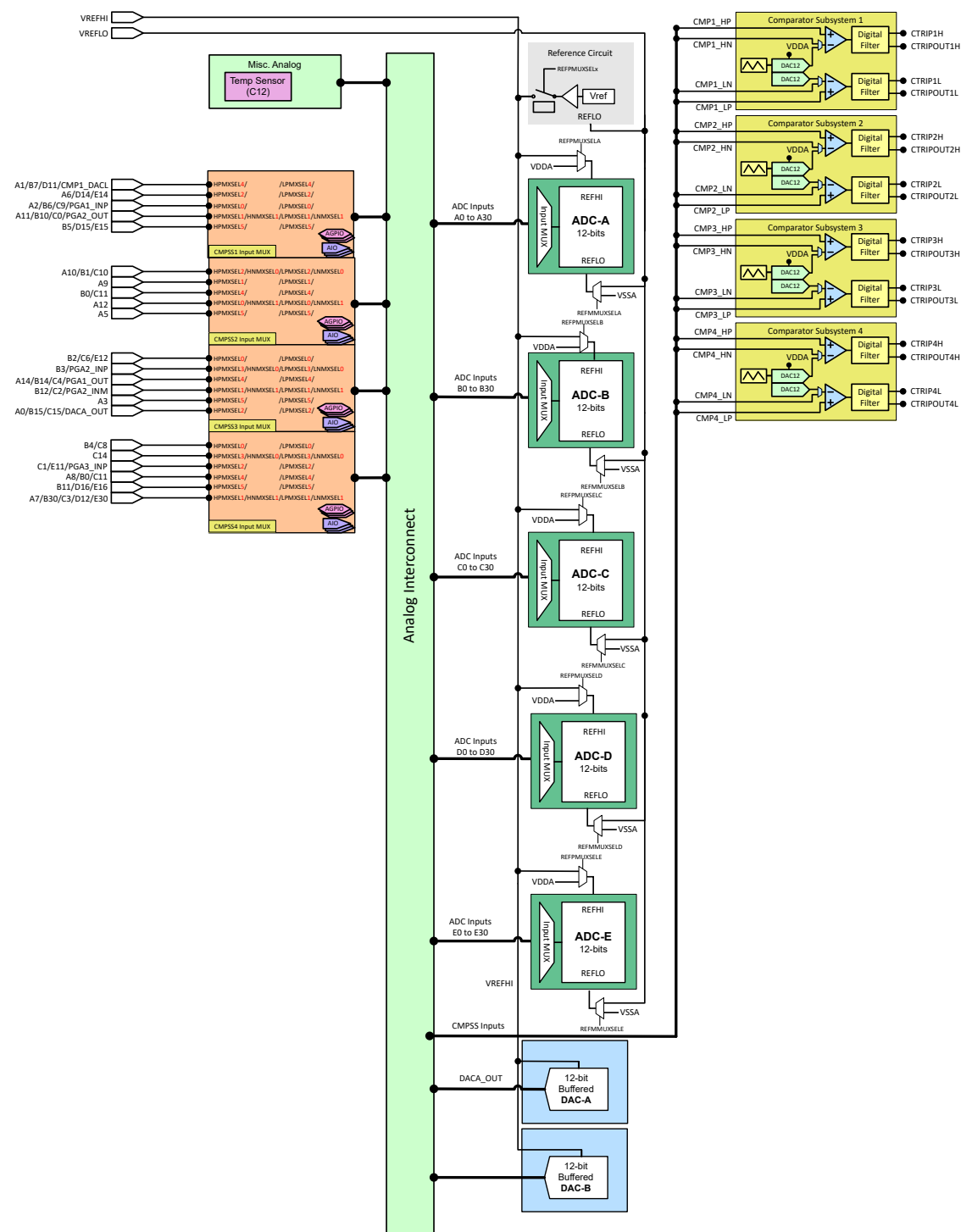
図 6-35. アナログサブシステムのブロック図 (100 ピン パッケージ)
